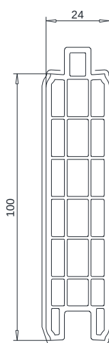
Lame de soubassement 110x24mm 109.361
