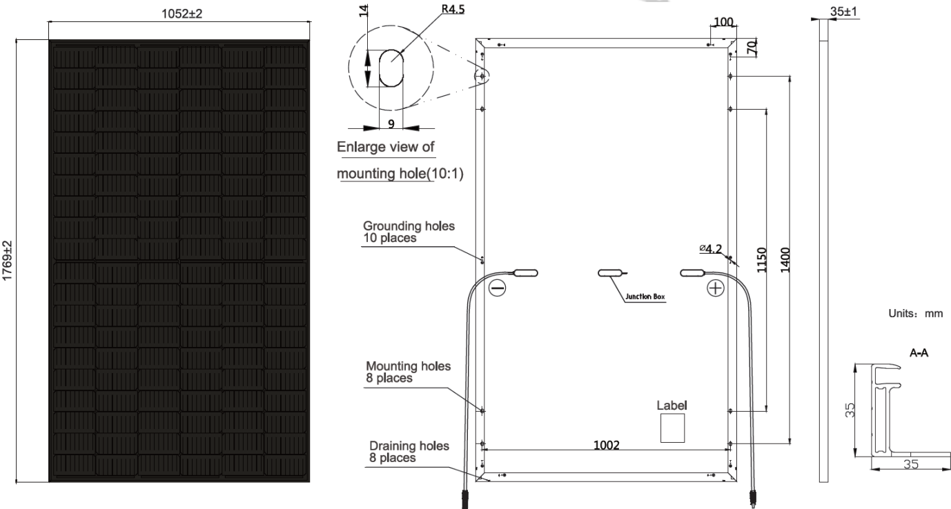
Modules photovoltaïques JA SOLAR JAM60S20/MR, JAM60S21/MR et son cadre
