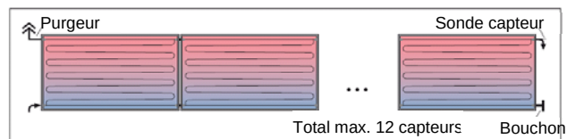
Champ de capteur raccordé cotés opposés
