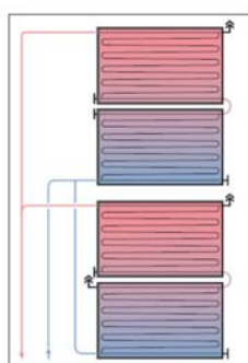
Champ de capteur raccordé même côté
