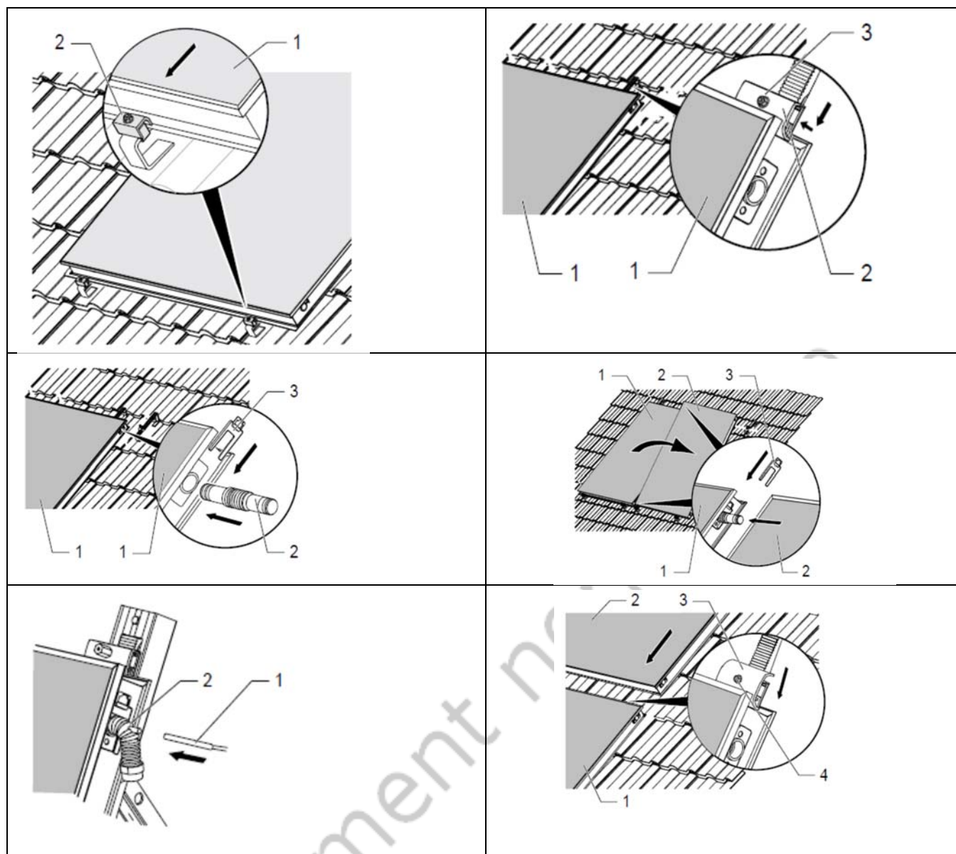
Figure 16 – Montage des capteurs.
