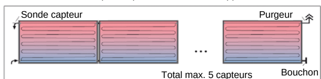
Champ de capteur raccordé même côté
