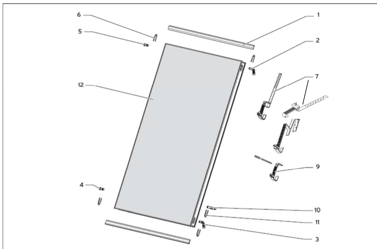
Figure 8 – Liste de matériel pour le montage sur toiture inclinée (cas d'un capteur).
