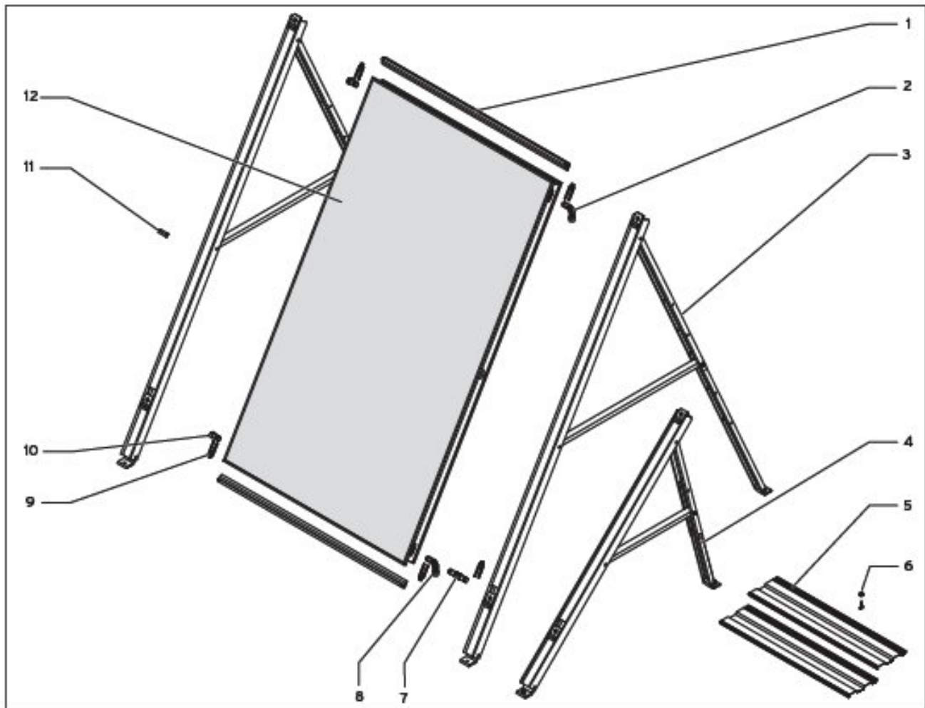
Figure 17 – Détail du kit de montage sur toiture plane.
