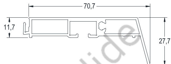
Capot ouvrant Z75 Réf : 32 918
