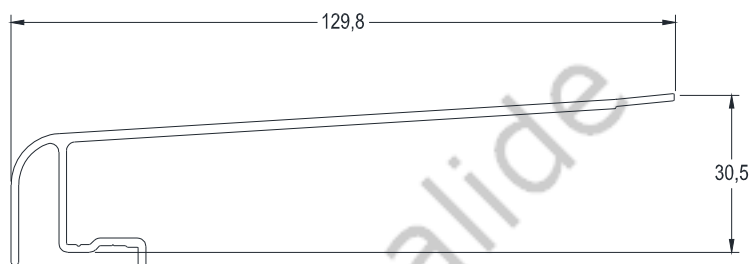
Joint capot dormant Réf : 126 201
