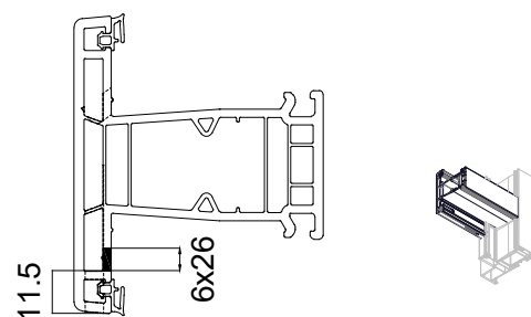
Equilibrage de pression Meneau
