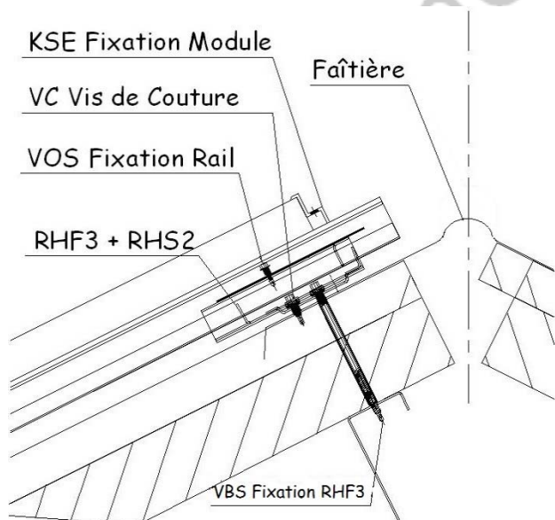
Figure 23 - Illustration de l'utilisation de la rehausse de faîtage (L'entretoise n'est pas représentée sur ces sections)
