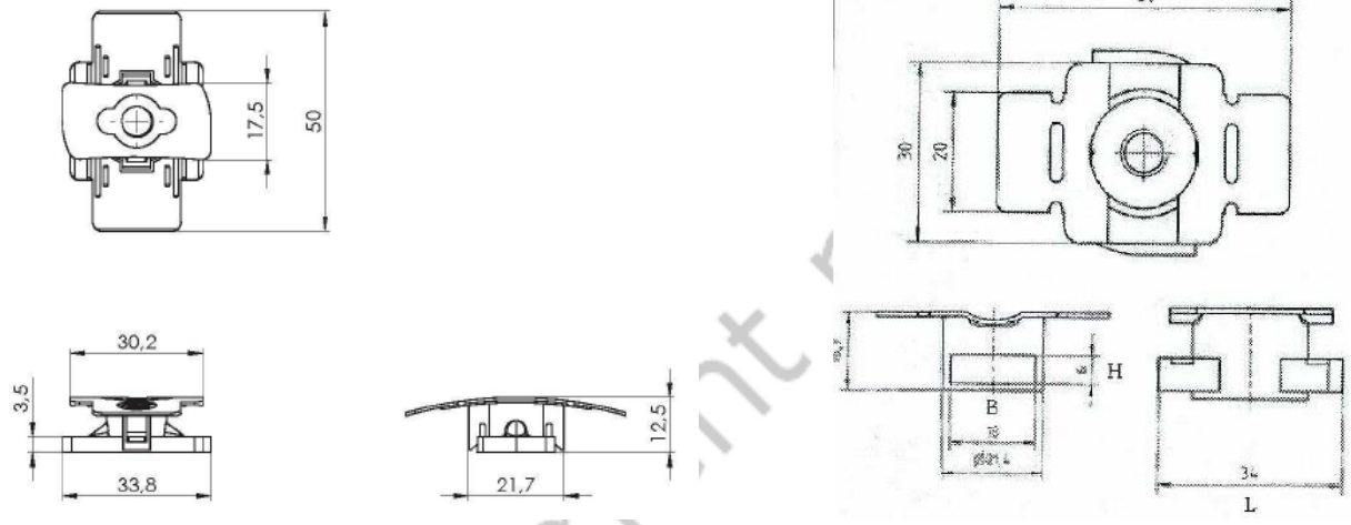
Écrous prisonniers
