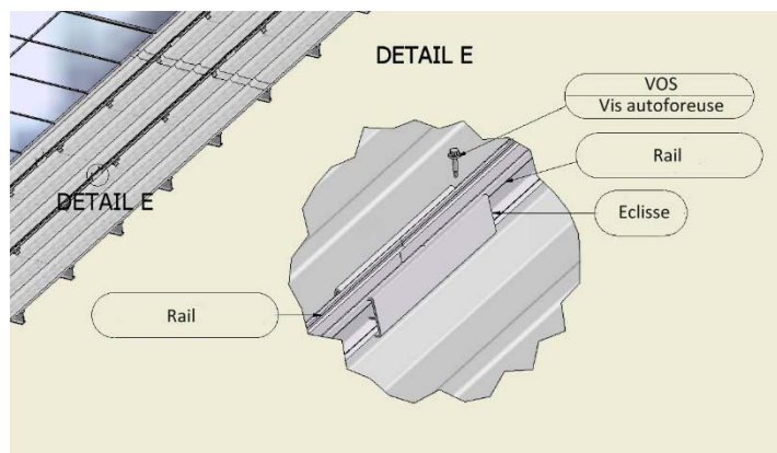
Figure 28 – Éclissage à la jonction de deux rails
