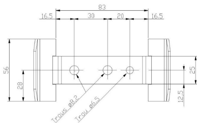
Figure 11 – Rehausse de faîtage
