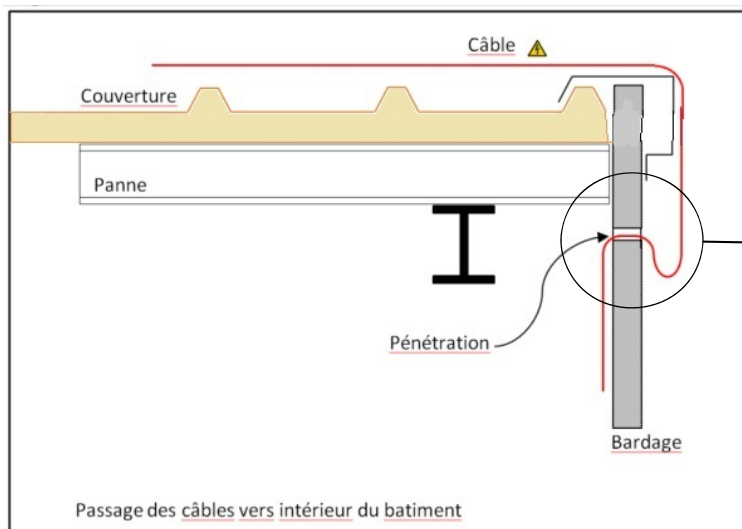
Figure 18 – Cheminement des câbles et exemple de passage des câbles à l'intérieur du bâtiment
