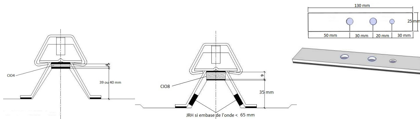
Figure 20 - Mise en place de la cale (L'entretoise n'est pas représentée sur ces sections)
