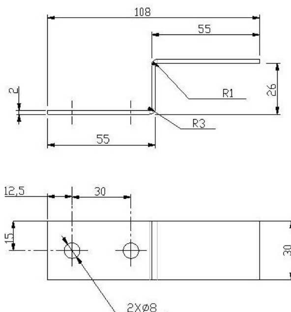
Figure 10 – Rehausse de blocage
