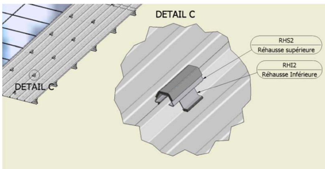
Figure 24 – Illustration de l'utilisation de la rehausse supérieure sur la rehausse inférieure
