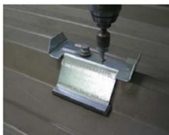
Figure 21 - Illustration de la fixation du perçage des panneaux sandwich et de la pose de l'entretoise (Cas simple vis ; pour le cas double vis voir Figure 25)
