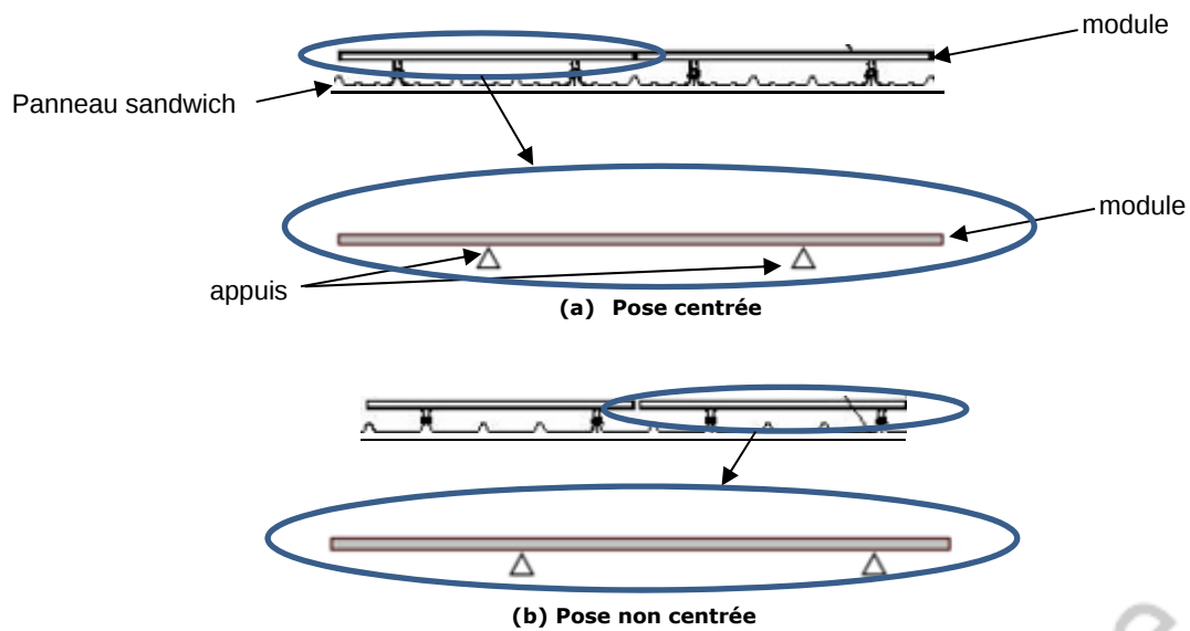
Figure 2 – Définition de pose des modules (a) "centrés" et (b) "non centrés"
