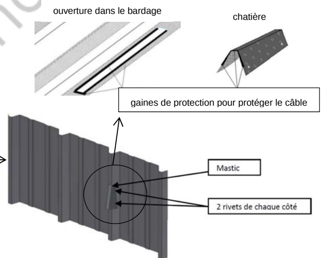
Exemple de cheminement des câbles
