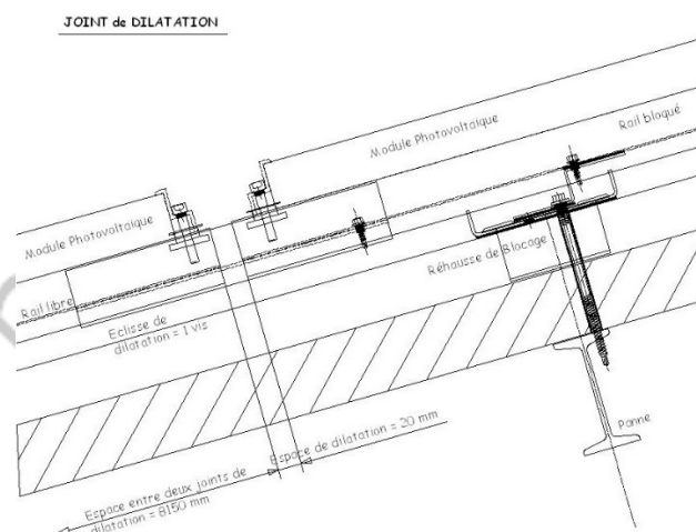
Figure 29 – Éclissage au joint de dilatation (L'entretoise n'est pas représentée sur ces sections)
