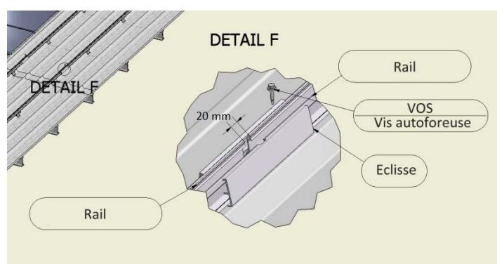
Figure 28 – Éclissage à la jonction de deux rails
