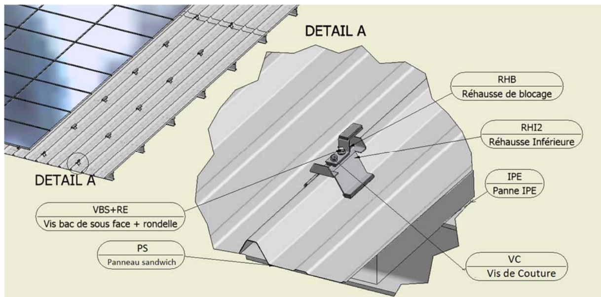
Figure 22 - Illustration de la fixation des panneaux sandwich à l'aide des rehausses inférieures avec la rehausse de blocage
