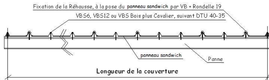
Figure 19 – Principe de répartition des fixations des panneaux sandwich
