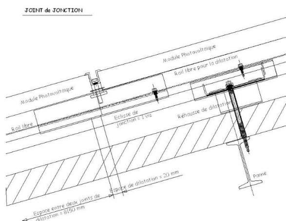
Figure 28 – Éclissage à la jonction de deux rails
