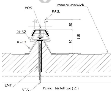
Figure 25 - Fixation du rail sur la rehausse de blocage ou la rehausse supérieure (L'entretoise n'est pas partout représentée sur ces sections)
