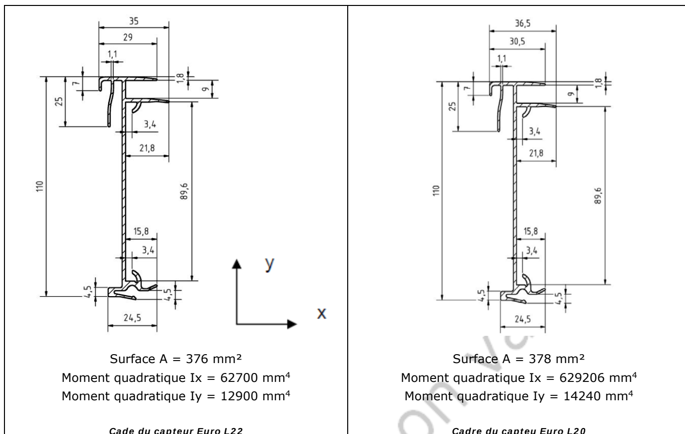
Figure 3.2 – Profilés du cadre du capteur.
