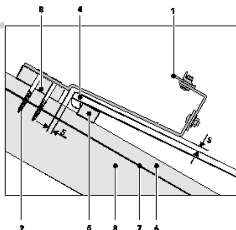
Figure 1.9 - Fixation pour tuiles à emboîtement ou à glissement à relief avec écran de sous-toiture.
