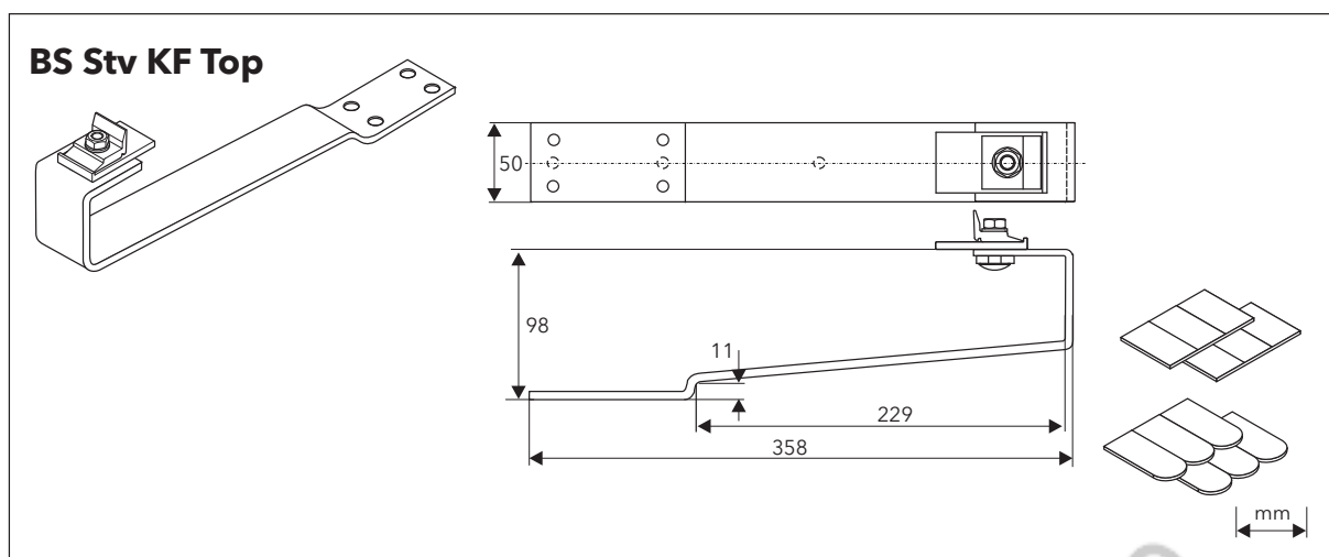
Patte de fixation BS Stv KF Top acier galvanisé - épaisseur moyenne de 6 mm
