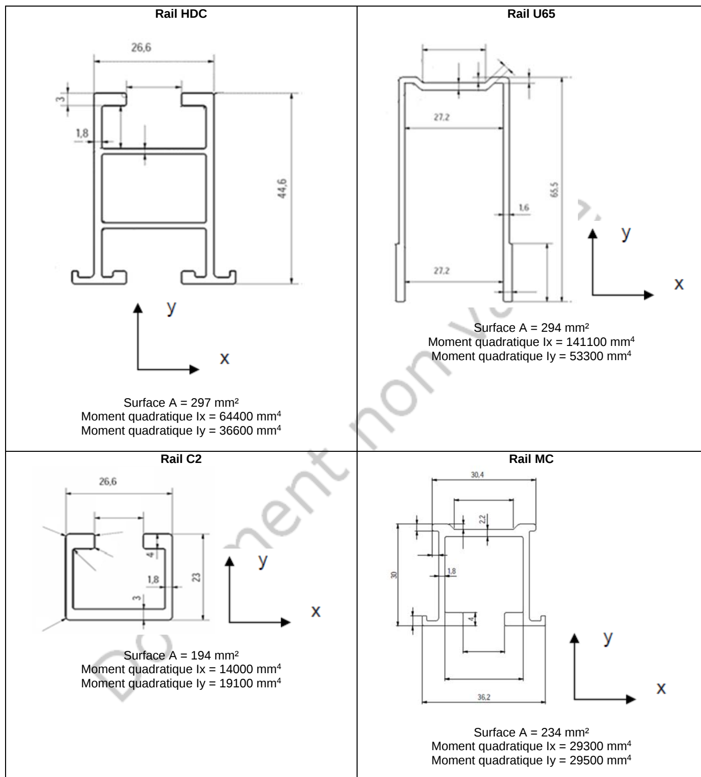
Figure 3.1 – Profilés du support incliné
