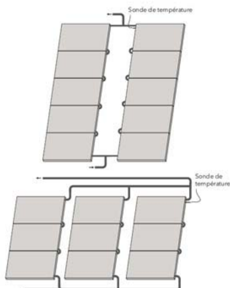
Figure 7 - Exemples de raccords des capteurs EURO L20AR / L22AR
