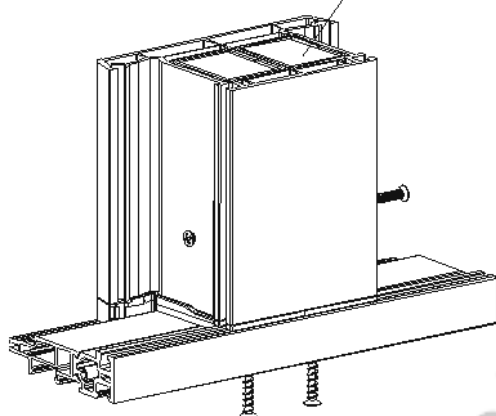
3-Vissages du meneau
