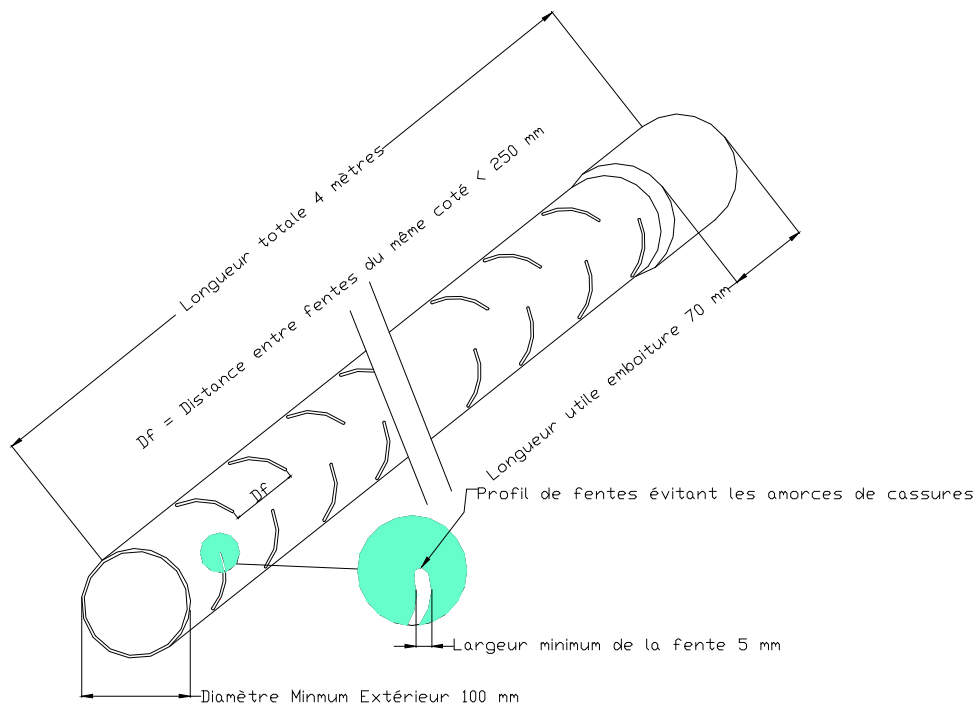
Figure 1 – Caractéristiques dimensionnelles des tubes OD.PRO Epandage
