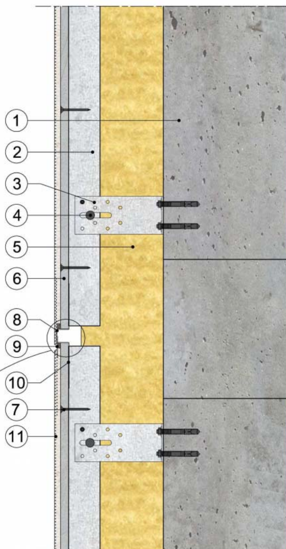
Figure 11 – Fractionnement de l'ossature acier bridée (longueur montant limitée à 6 m)
