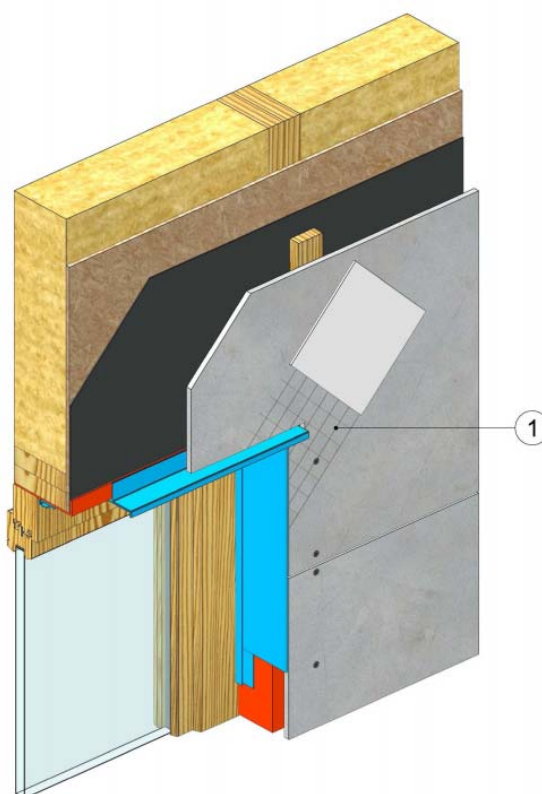
Figure 5b – Pose sur COB Etape 1 : Disposition des plaques Aquapanel – Détail d'angle
