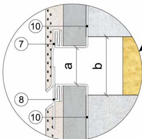
Figure 11 – Fractionnement de l'ossature acier bridée (longueur montant limitée à 6 m)
