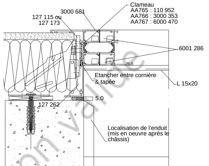
Coupe horizontale AA765 kalory Cas caillebotis
