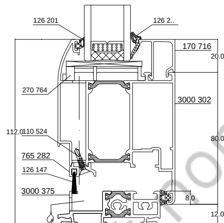
Traverse basse avec seuil PMR
