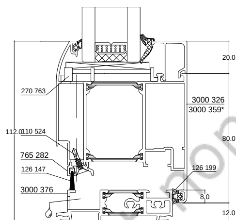
Traverse basse avec seuil PMR
