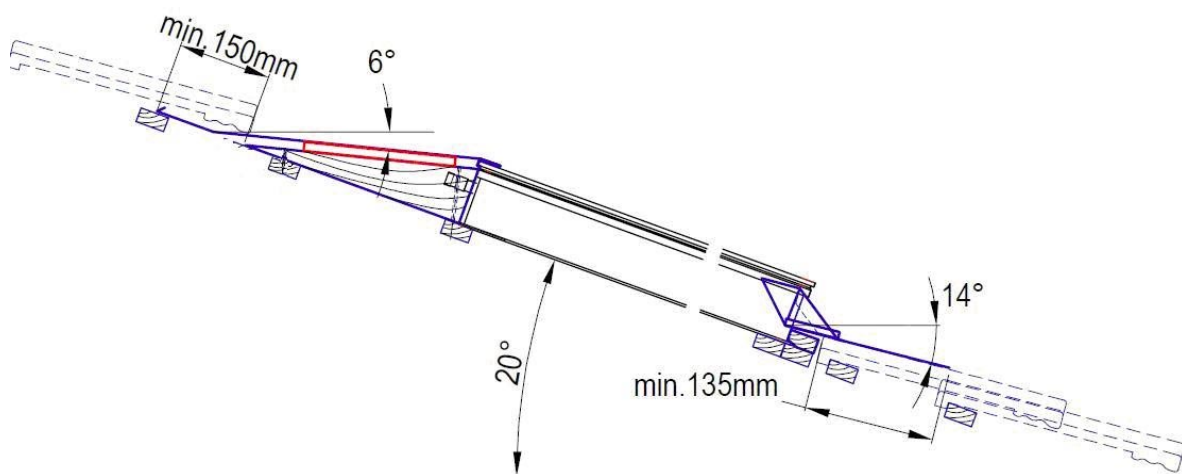
Figure 1.9 - Recouvrements minimaux des éléments de couverture en amont et en aval des capteurs et pentes résiduelles pour une pente de 20° - Tuiles à emboîtement ou à glissement à relief.
