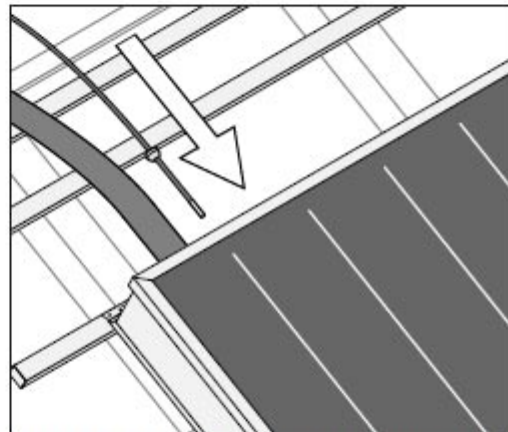
Fig. 18 Insérez la sonde de température dans le doigt de gant, glissez le câble dans le passe-câble en caoutchouc, refermez l'ouverture. Faites passer le câble sous la toiture.
