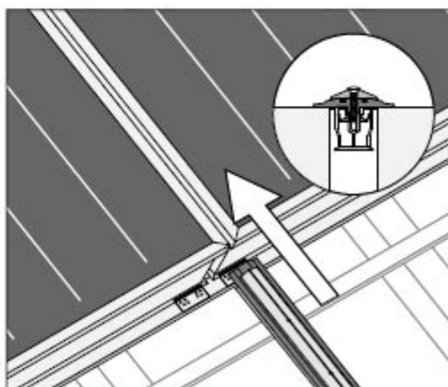
Fig. 14 Glissez le rail d'étanchéité prémonter entre les deux capteurs, rapprochez les capteurs et vissez le rail par le dessus.
