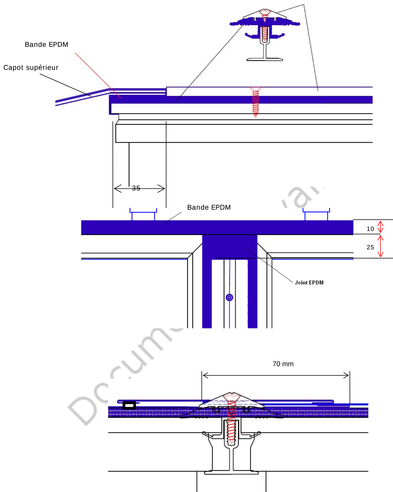
Figure 1.12 – Détail de la jonction des bavettes supérieures avec le joint intercapteur.
