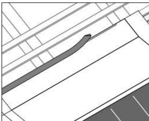
Fig. 33 Collez une bande de caoutchouc mousse sur le capot supérieur le long de la pliure.
