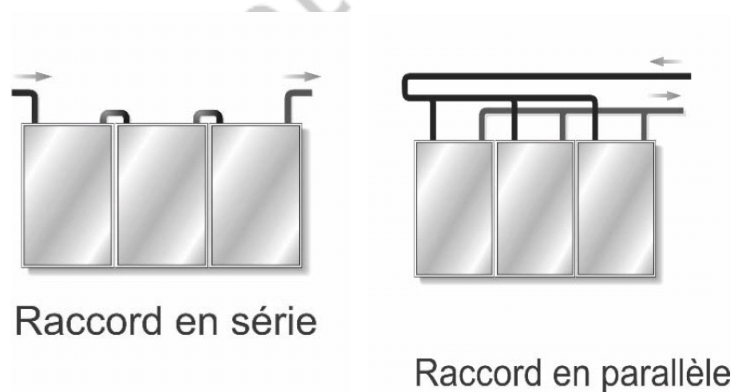
Figure 6 - Exemples de raccordements des capteurs EURO C20 / C22.
