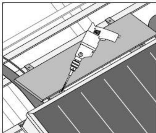
Fig. 18 Posez le support en bois contre le capteur et fixez-le avec les vis à bois 4 x 35 et 5 x 120
