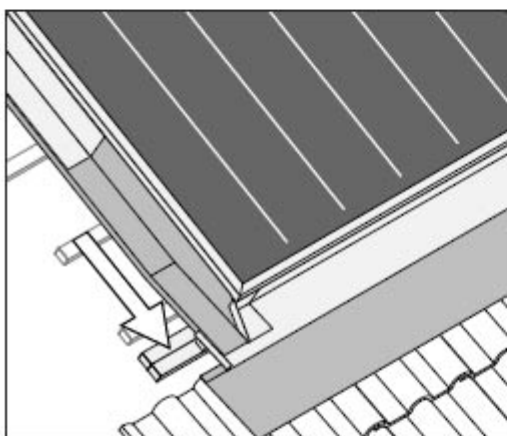
Fig. 23 Faites coulisser la bavette inférieure jusqu'à ce qu'elle vienne s'emboîter dans le rabat de la cornière inférieure.
