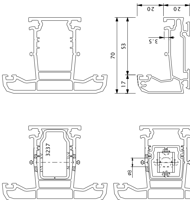
ASSEMBLAGE MECANIQUE DU MENEAU 3082 sur seuil DK ZD
