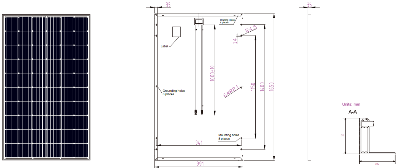
Modules photovoltaïques et cadre : JAM60S01-XXX/PR
