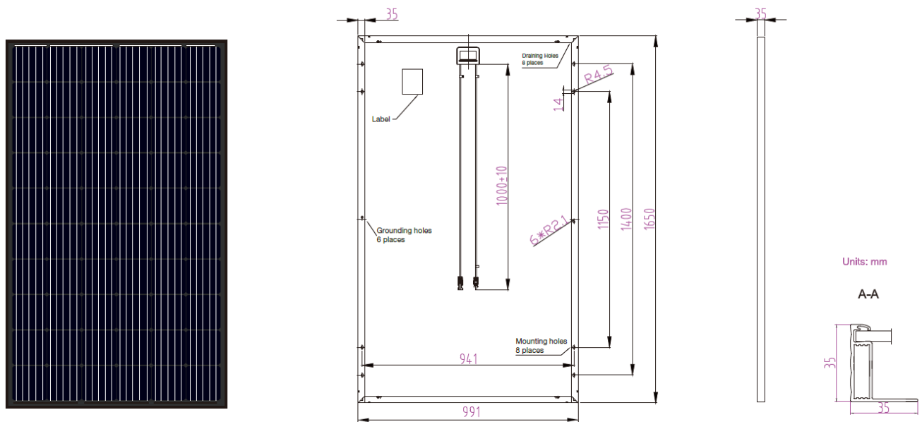
Modules photovoltaïques et cadre : JAM60S02-XXX/PR
