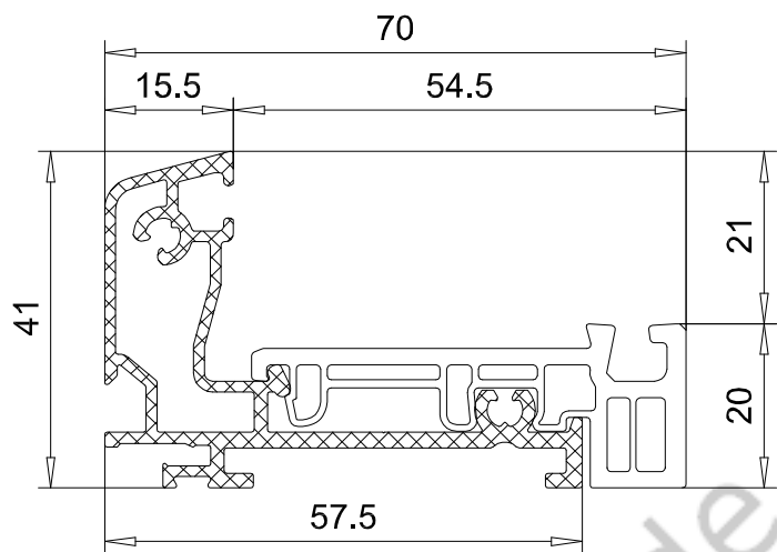
Seuil à rupture de pont thermique 104.286
