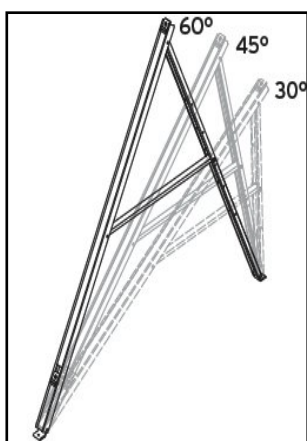
Figure 19 – Détails de la mise en œuvre d'un bâti.
