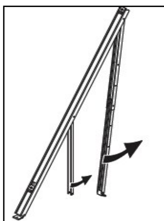
Figure 20 – Mise en œuvre des châssis par vissage direct dans la structure du bâtiment (plots béton).
