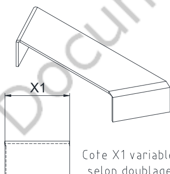
Capot d'écarteur
