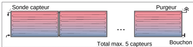
Champ de capteur raccordé même coté
