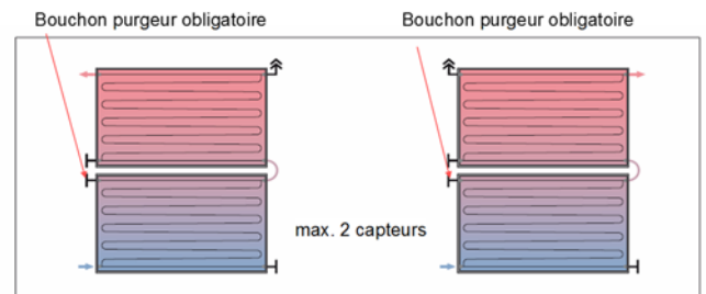
Champ de capteur horizontaux montés en champ vertical (maxi 2)
