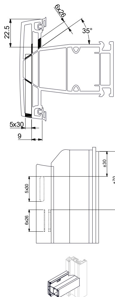
Traverse Intermédiaire d'ouvrant
