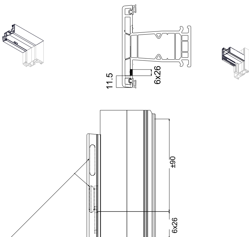
Equilibrage de pression Meneau
