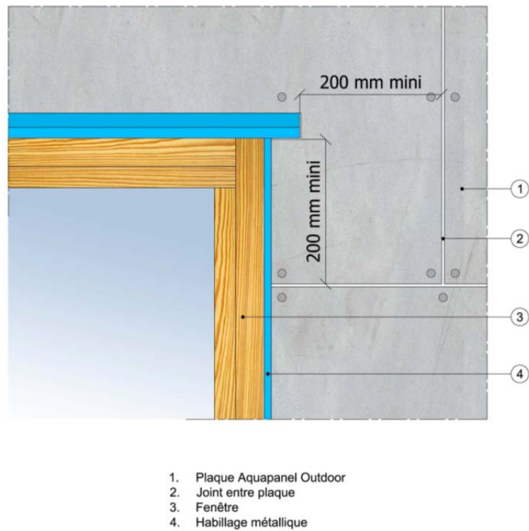
Figure 10b – Pose sur COB Etape 1 : Disposition des plaques Aquapanel – Détail d'angle
