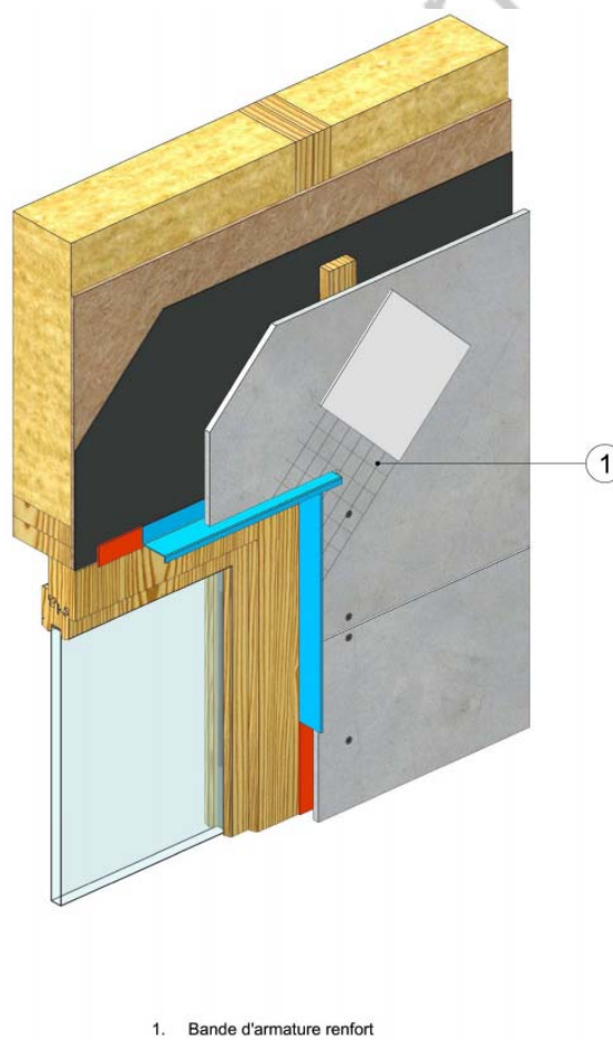
Figure 10c – Pose sur COB – Perspective linteau Etape 2 : Mise des renforcements des ouvertures
