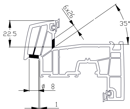
Drainages ouvrant
