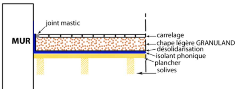
Figure 6 – Joint mastic en périphérie pour local E2
