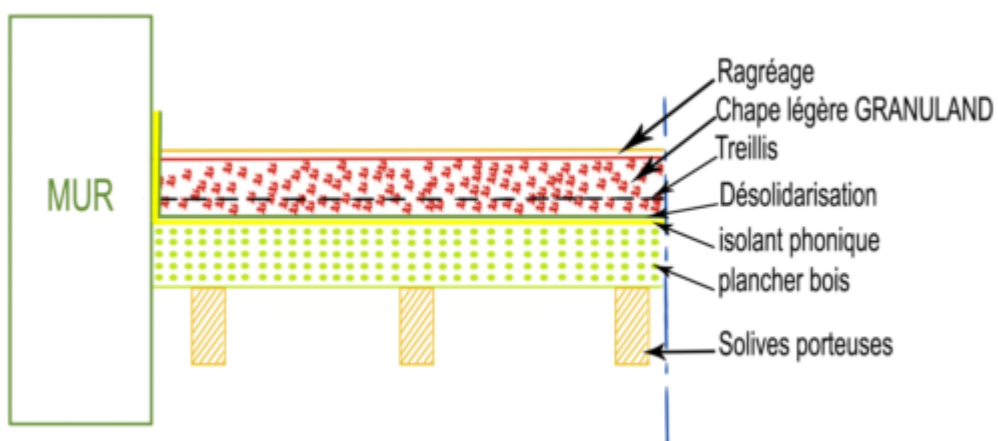
Figure 5 – Chape flottante sur isolant phonique
