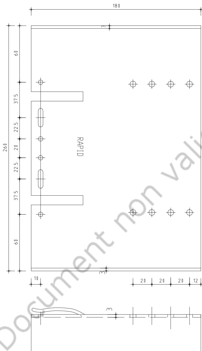
Figure 5 – Rallonge pour étrier NFT 240 mm
