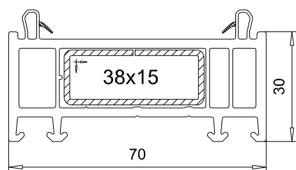
Elargisseur 30mm
