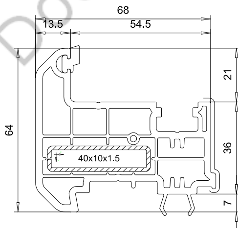
Battement rapporté 64mm
