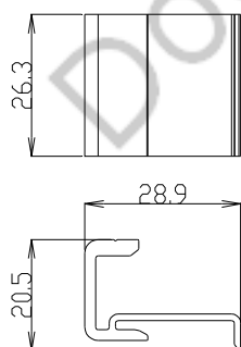
Cale de réglage renfort vertical Réf 49903
