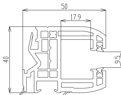
Coulisse U4
