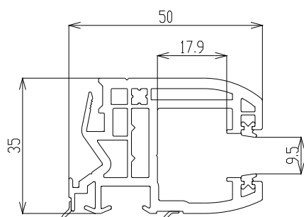
Coulisse U3
