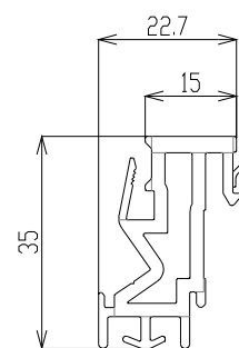
Elargisseur EL
