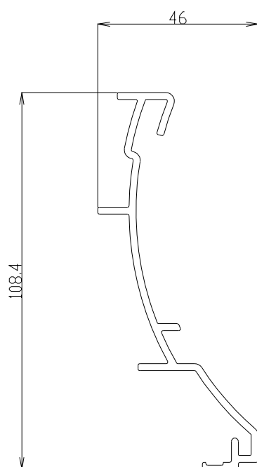
Renfort vertical BLOC Réf 49902
