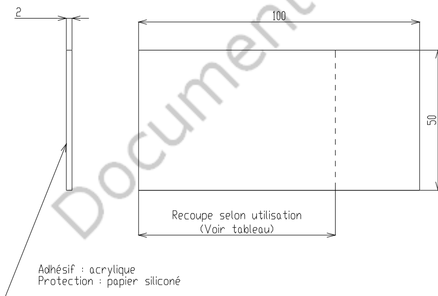
Etanchéité Coulisse / Pièce d'appui
