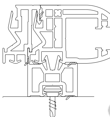
Etanchéité Coulisse / Pièce d'appui
