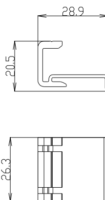
Cale renfort vertical Réf 49904
