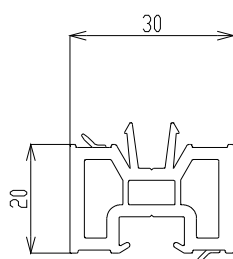
Réhausse RE
