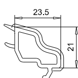
Parcloses 107.226 Vitrage: 24 ¼
