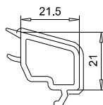
Parcloses 107.224 Vitrage: 26 ¼
