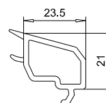
Parcloses 107.244 Vitrage: 24 ¼
