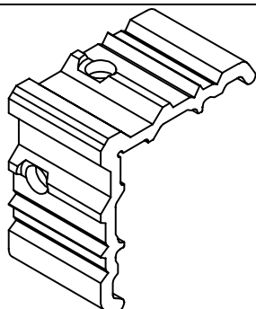
EM002 Equerre à sertir Chambre 10 x 43
