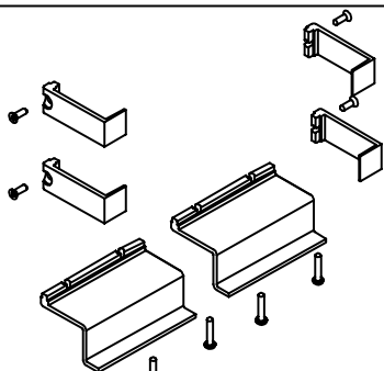
CM022 Pièce de sécurité italienne TV
