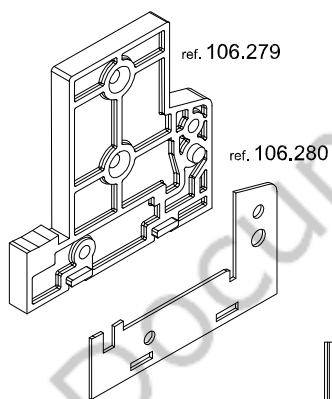
Embout seuil filant réversible 106.279 Joint 106.280
