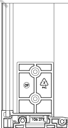
Embout seuil filant réversible 106.277 Joint 106.278
