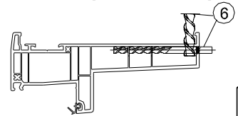
Variante perçage 1
