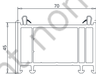
Elargisseur 45mm 114.202.2
