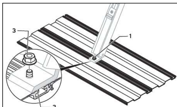
Boulonnage des bâtis sur les plaques
