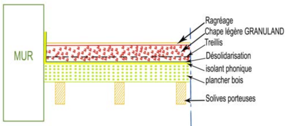
Figure 5 – Chape flottante sur isolant phonique
