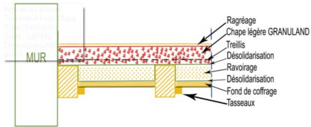
Figure 1 – Coffrage porteur entre solives
