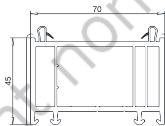
Elargisseur 45mm 114.202.2
