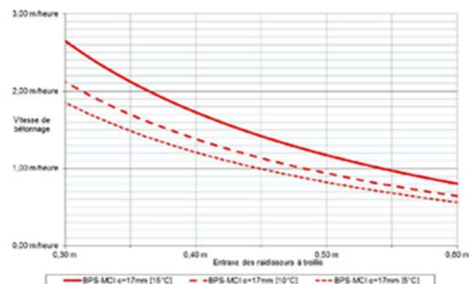
Vitesse de bétonnage pour les BPS en fonction de la température et de l'entraxe des raidisseurs (pour un enrobage du treillis C_{imin} = 17mm )
