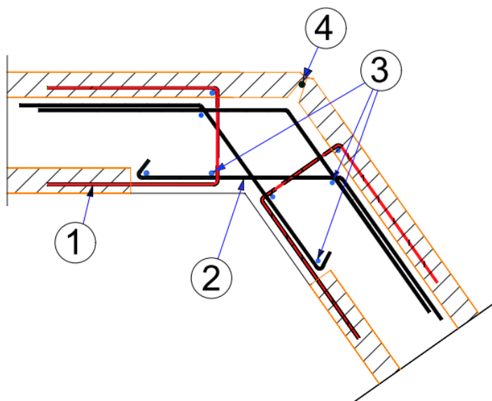
c) Configurations pour un angle supérieur à 45°
