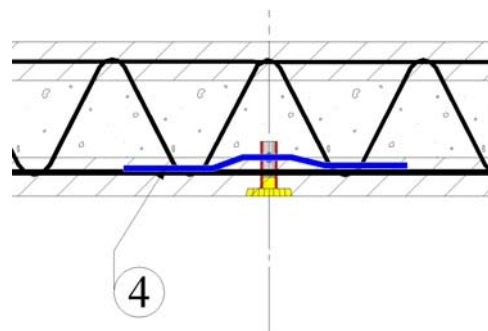
b) Coupe verticale sur douille métallique
