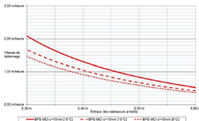
Vitesse de bétonnage pour les BPS en fonction de la température et de l'entraxe des raidisseurs (pour un enrobage du treillis C_{imin} = 15mm )
