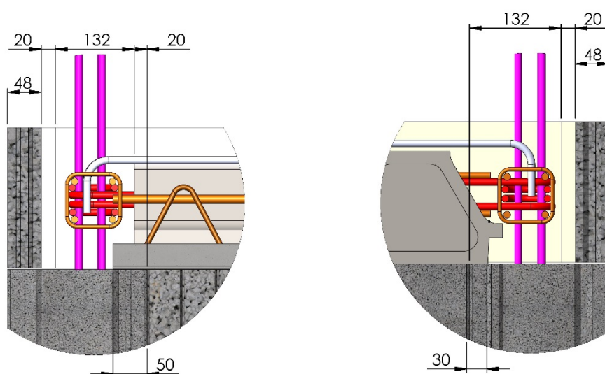
Figure 12 Coupe d'un plancher avec la planelle « ISOPLANEL »
