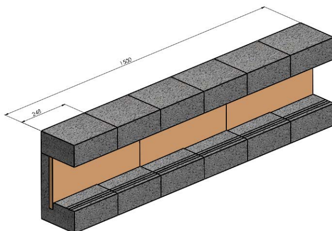
Figure 8 Principe de montage des planelles « RUPTHERM »
