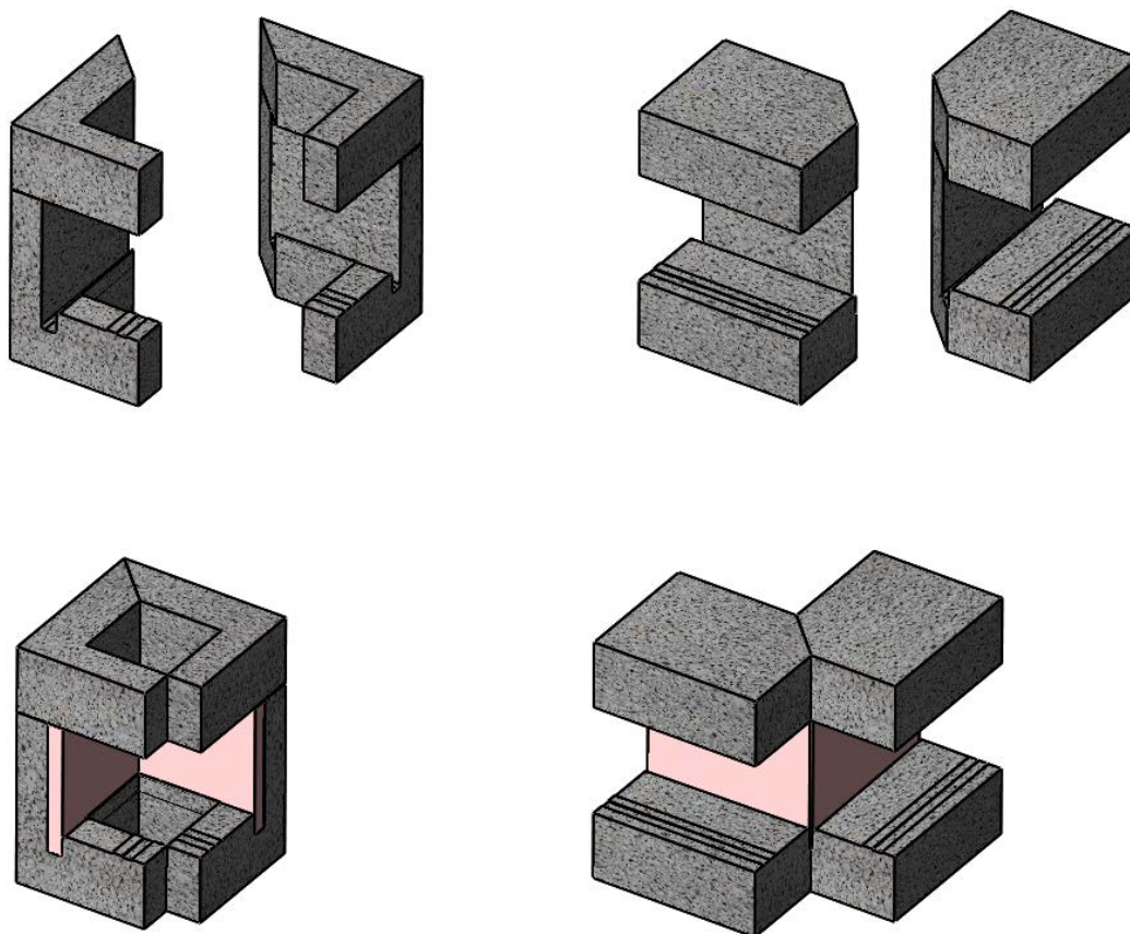
Figure 18 Réalisation des points singuliers des « RUPTHERM »
