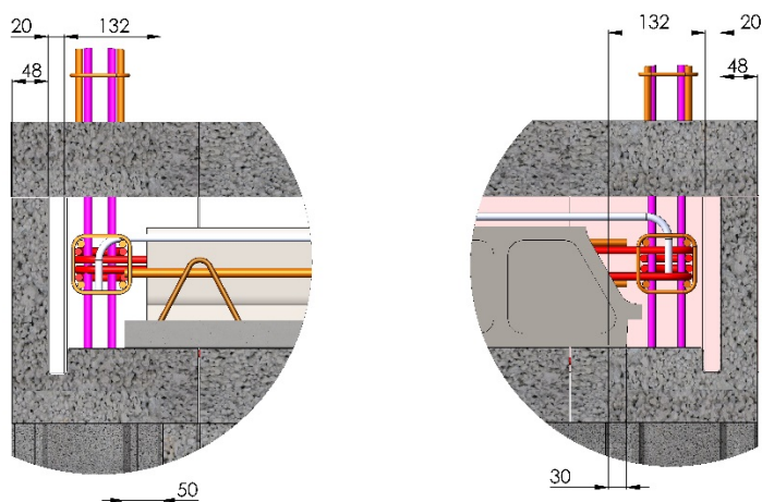
Figure 16 Coupe d'un plancher avec la planelle « RUPTHERM »
