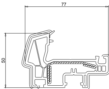
Battelement monobloc fenêtre 103.338
