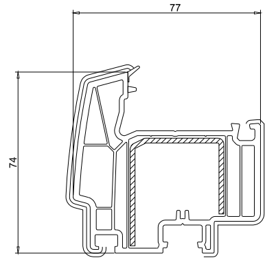
Battelement monobloc ouvrant serrure 103.336
