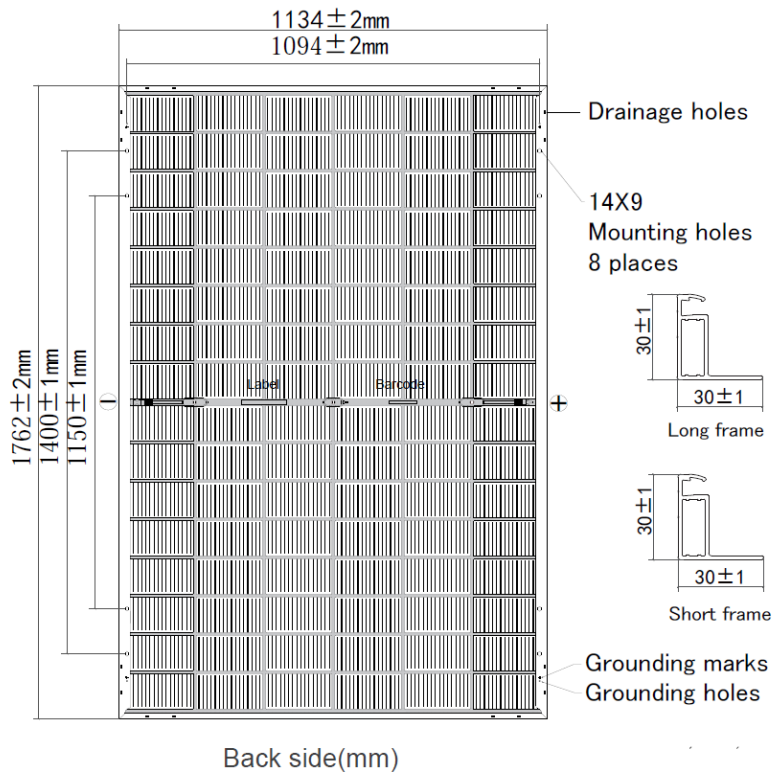
Modules DMEGC DMxxxG12RT-B48HSW/HBW/HBB/HBT (cadre 30x30)
