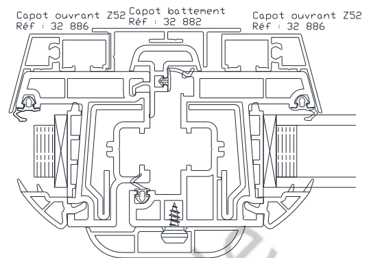
Ouvrant Z52
