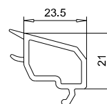
Parcloses 107.244 Vitrage: 24 ¼
