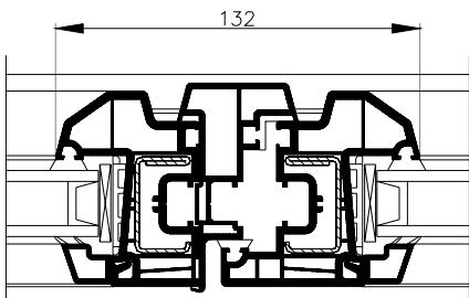
Battée: art: 541140 Ouvrant Z52: art: 554101
