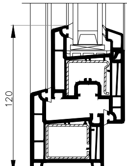
Dormant de 68: art: 554041 Ouvrant Z60: art: 554051
