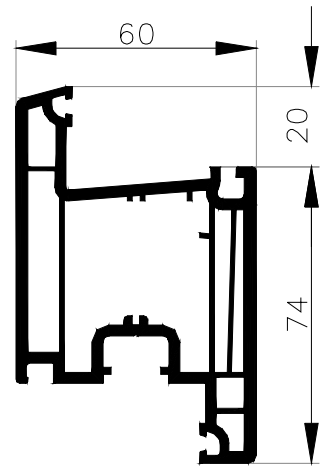
Ouvrant Z 74 Art: 554081
