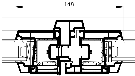
Battée: art: 541140 Ouvrant Z60: art: 554051
