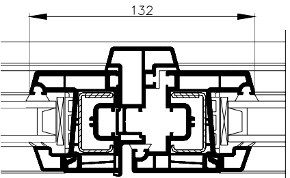
Battée: art: 541140 Ouvrant Z52: art: 554141
