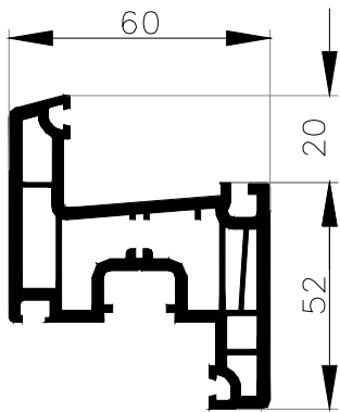
Ouvrant Z 52 Art: 554141
