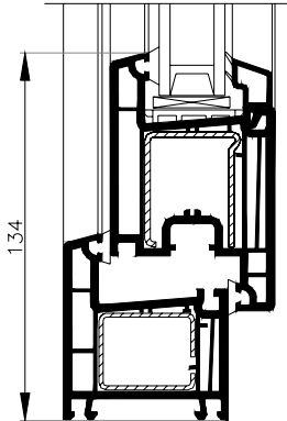
Dormant de 68: art: 554041 Ouvrant Z74: art: 554081
