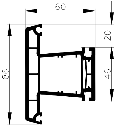
Meneau de 86 Art: 554091
