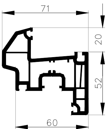
Ouvrant Z 52 Art: 554101
