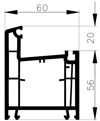
Dormant de 76 Art: 554061
