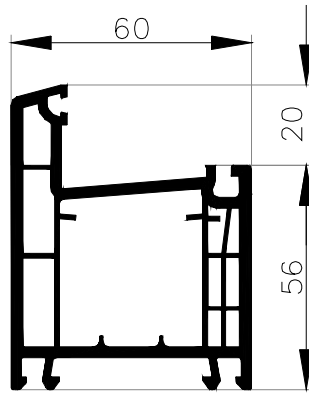
Dormant de 76 Art: 554121
