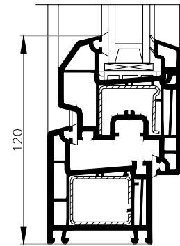
Dormant de 68: art: 554041 Ouvrant Z60: art: 554111
