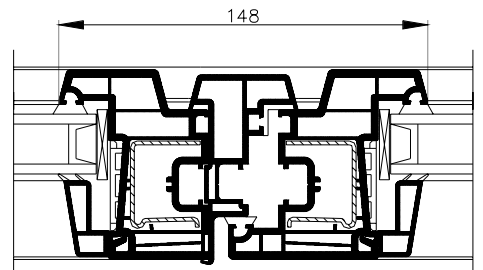
Battée: art: 541140 Ouvrant Z60: art: 554071
