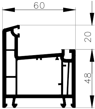
Dormant de 68 Art: 554041
