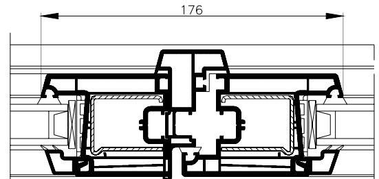
Battée: art: 541140 Ouvrant Z74: art: 554081
