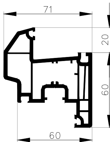
Ouvrant Z 60 Art: 554111
