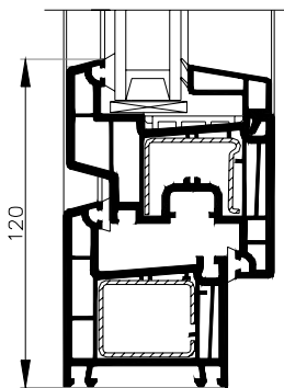
Dormant de 68: art: 554041 Ouvrant Z60: art: 554071
