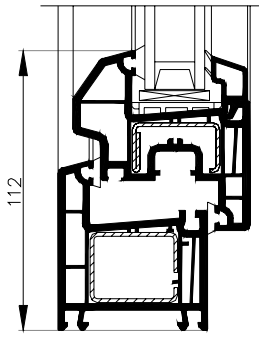
Dormant de 68: art: 554041 Ouvrant Z52: art: 554101
