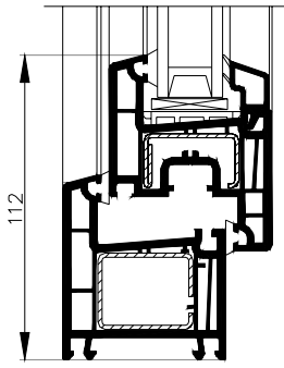
Dormant de 68: art: 554041 Ouvrant Z52: art: 554141
