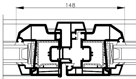
Battée: art: 541140 Ouvrant Z60: art: 554111
