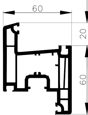
Ouvrant Z 60 Art: 554051
