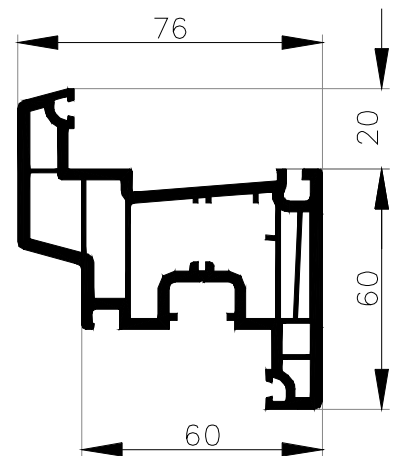
Ouvrant Z 60 Art: 554071
