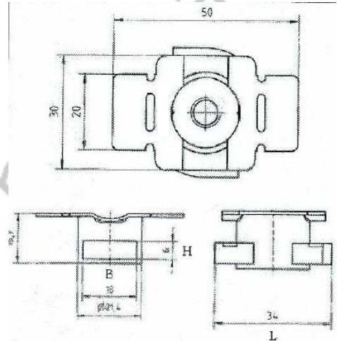
Écrous prisonniers
