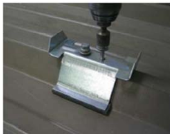
Figure 21 - Illustration de la fixation du perçage des panneaux sandwich et de la pose de l'entretoise (Cas simple vis ; pour le cas double vis voir Figure 25)
