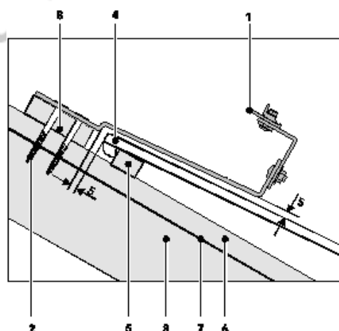
Figure 1.9 - Fixation pour tuiles à emboîtement ou à glissement à relief avec écran de sous-toiture.
