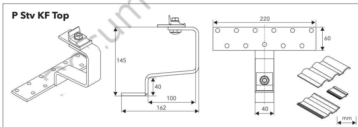
Figure 1.5 - Pattes de fixations : tuiles à relief – acier galvanisé.
