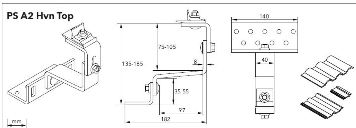
Figure 1.3 - Pattes de fixations : tuiles à relief – acier inoxydable.
