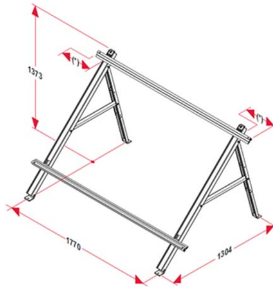
Figure 18 – Dimension du champ de captage.
