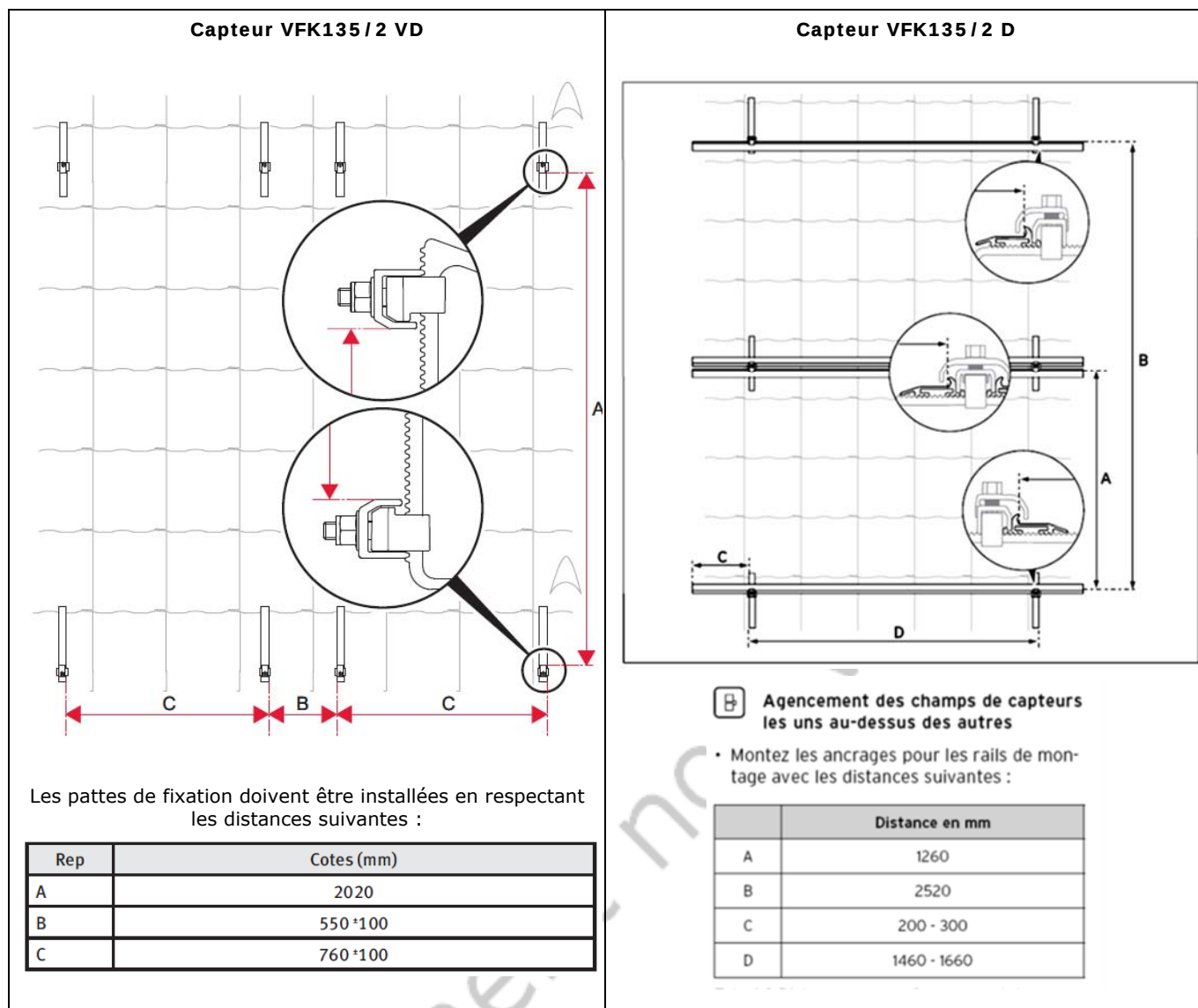
Figure 10 – Agencement des capteurs.
