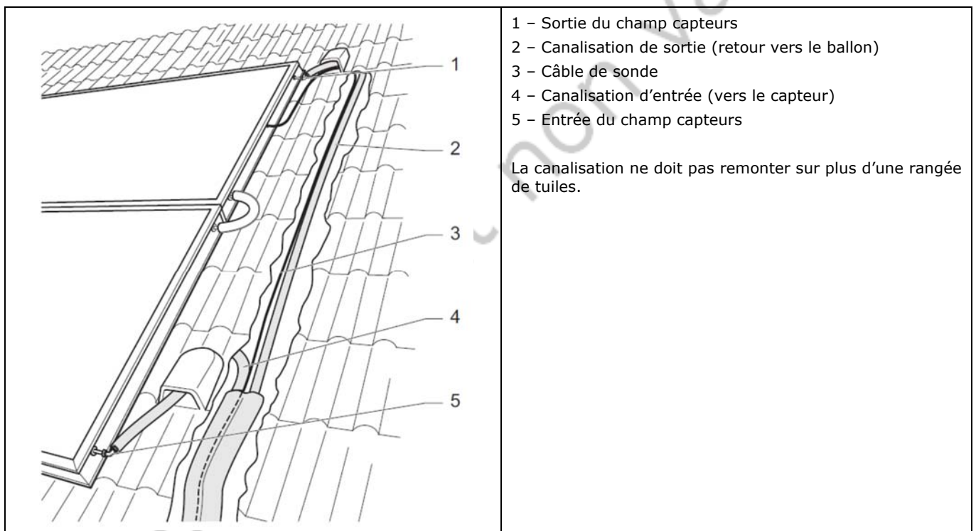
Figure 7 – Passage des canalisations au travers de la couverture.
