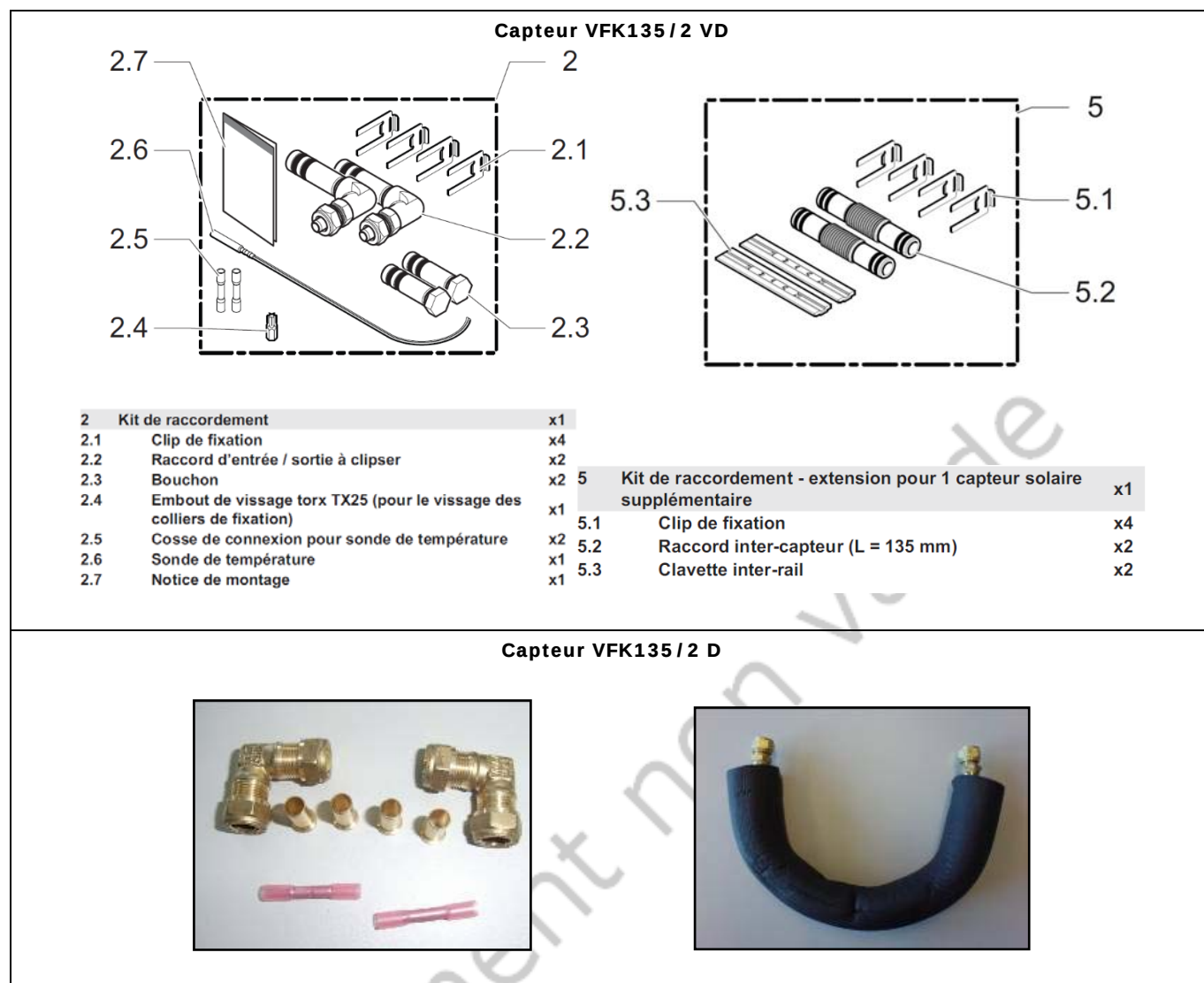
Figure 5 - Raccords hydrauliques et manchons thermo rétractables pour raccordement de la sonde.
