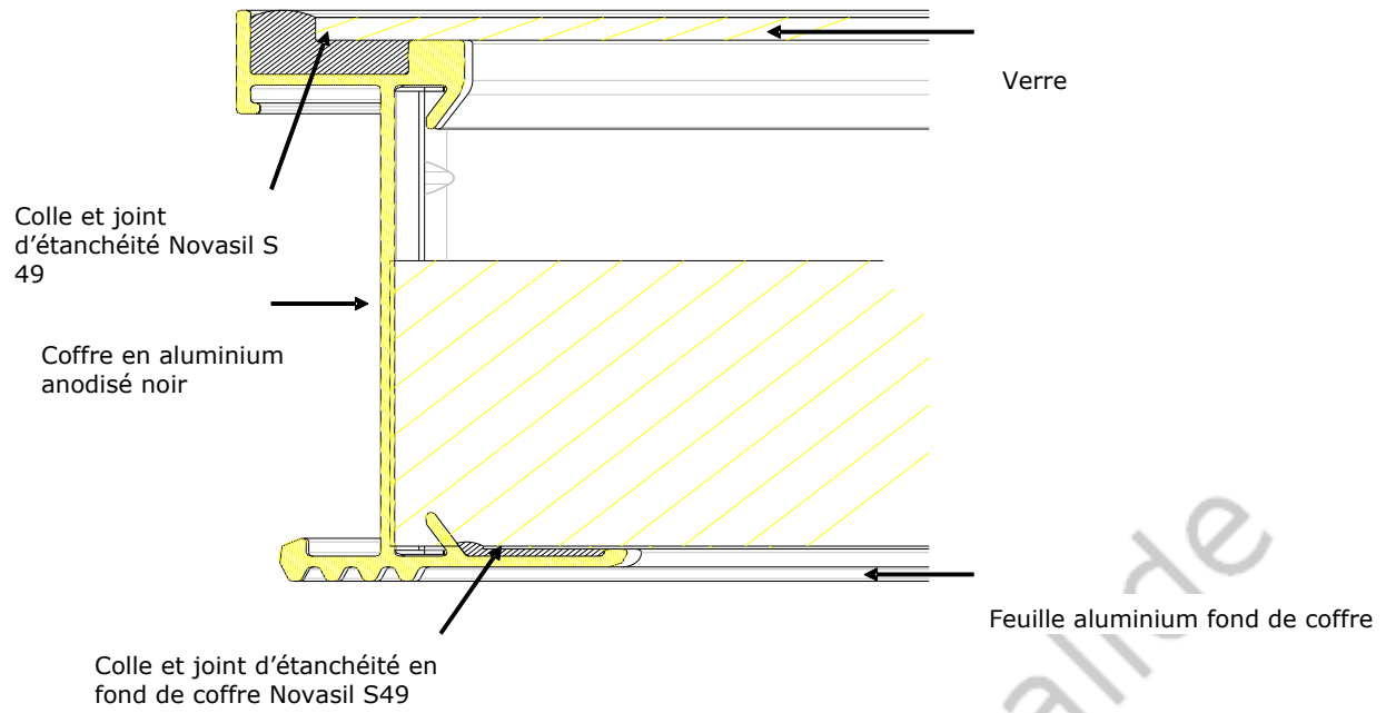
Figure 2 – Vue en coupe du coffre.
