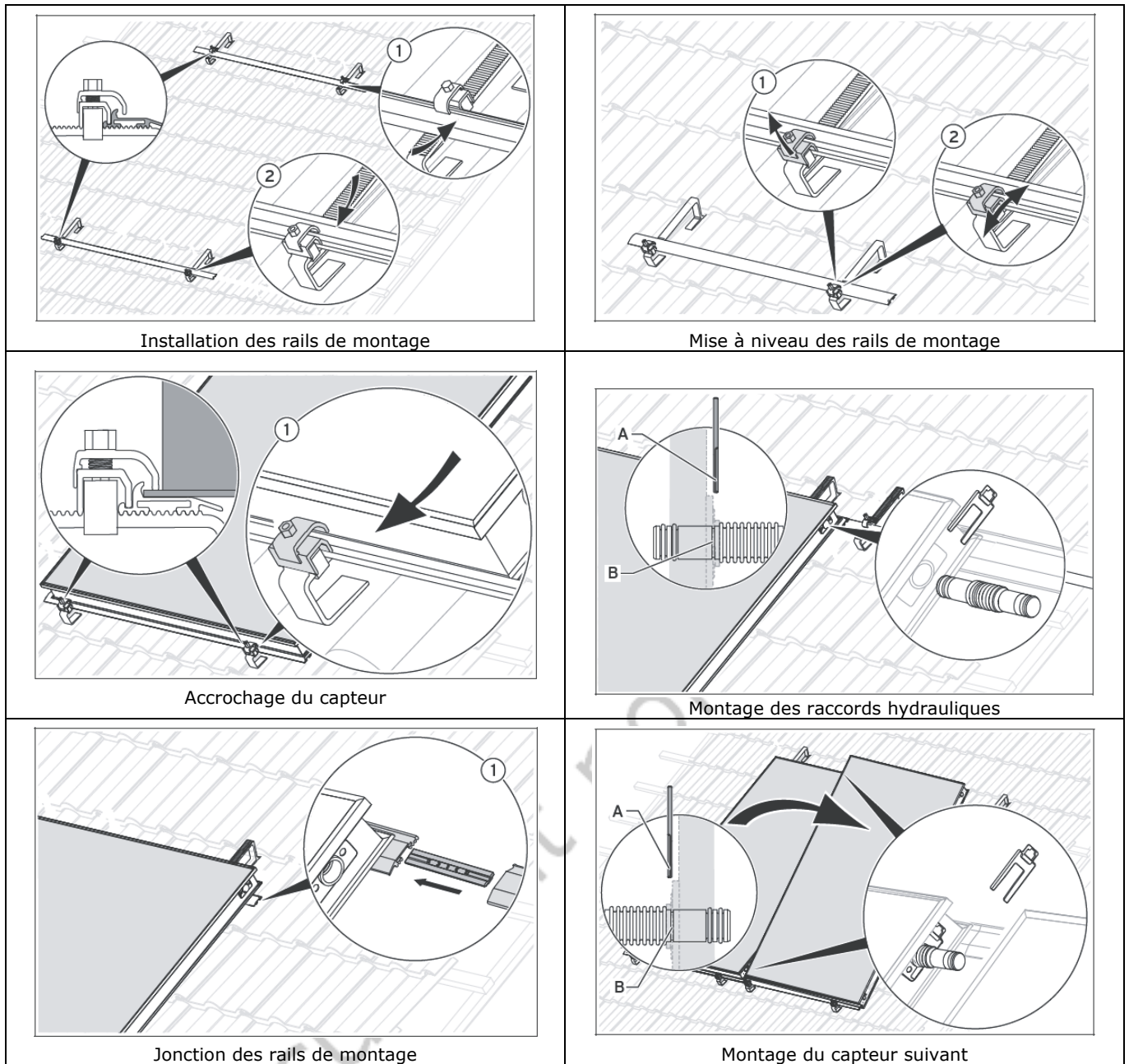
Figure 16 – Montage des capteurs.
