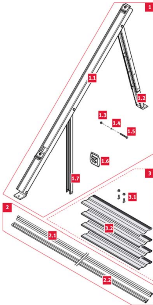
Figure 17 – Détail du kit de montage sur toiture plane.
