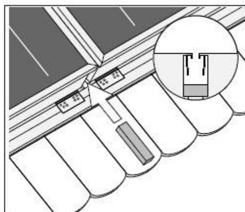
12 Ajustez la distance entre les capteurs à 35 mm à l'aide des bords en bois.
