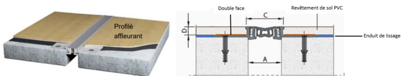
Figure 1 : Exemples de profilés de recouvrement de joints de dilatation
