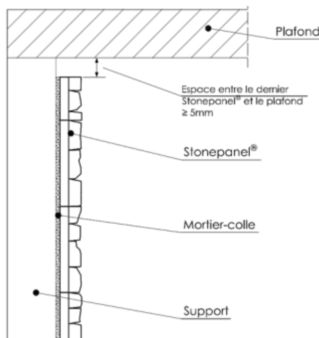
Figure 5b – Mise en œuvre de STONEPANEL en murs intérieurs
