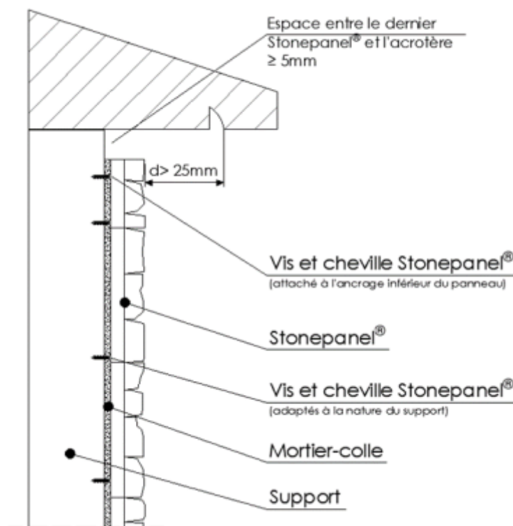
Figure 10 – Arêtes supérieures
