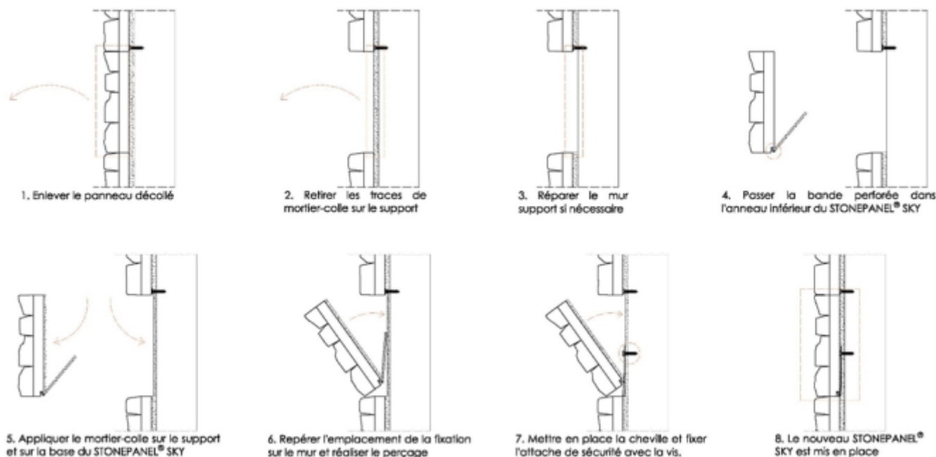
Figure 14b – Installation avec attache intérieure
