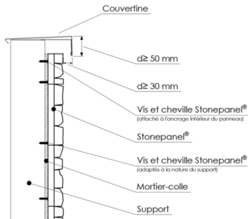
Figure 11 – Dessus d'acrotère
