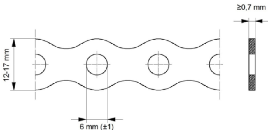
Figure 3 – Élément de sécurité : bande perforée
