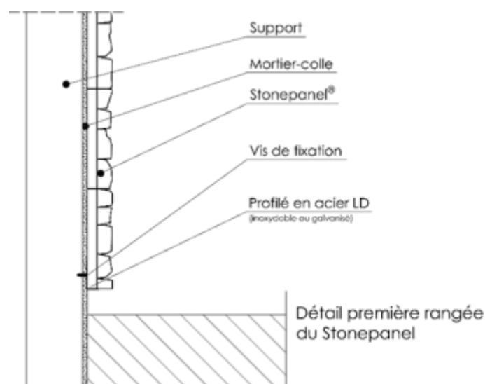
Figure 4b – Mise en œuvre avec un profilé en métal en intérieur
