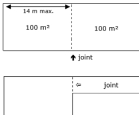
Figure 1 - Joint de fractionnement
