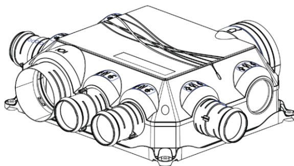
Figure 39 – Groupes d'extraction VENTILIS BC+
