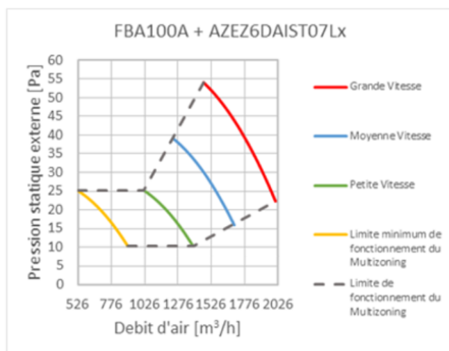
Figure 7 – Unité intérieure FBA100A Courbes débit/pression
