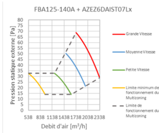
Figure 8 – Unités intérieures FBA125A et FBA140A Courbes débit/pression
