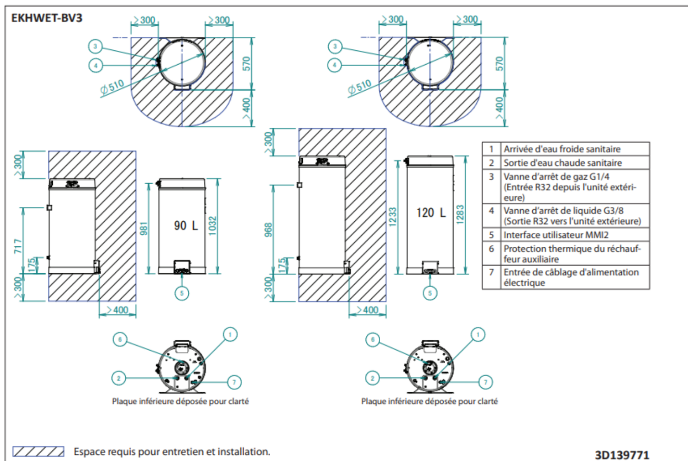
Figure 3 – Ballon mural ECS 90 / 120 L – visuel et caractéristiques dimensionnelles
