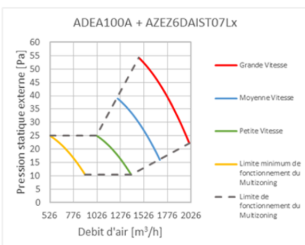
Figure 11 – Unité intérieure ADEA100A Courbes débit/pression
