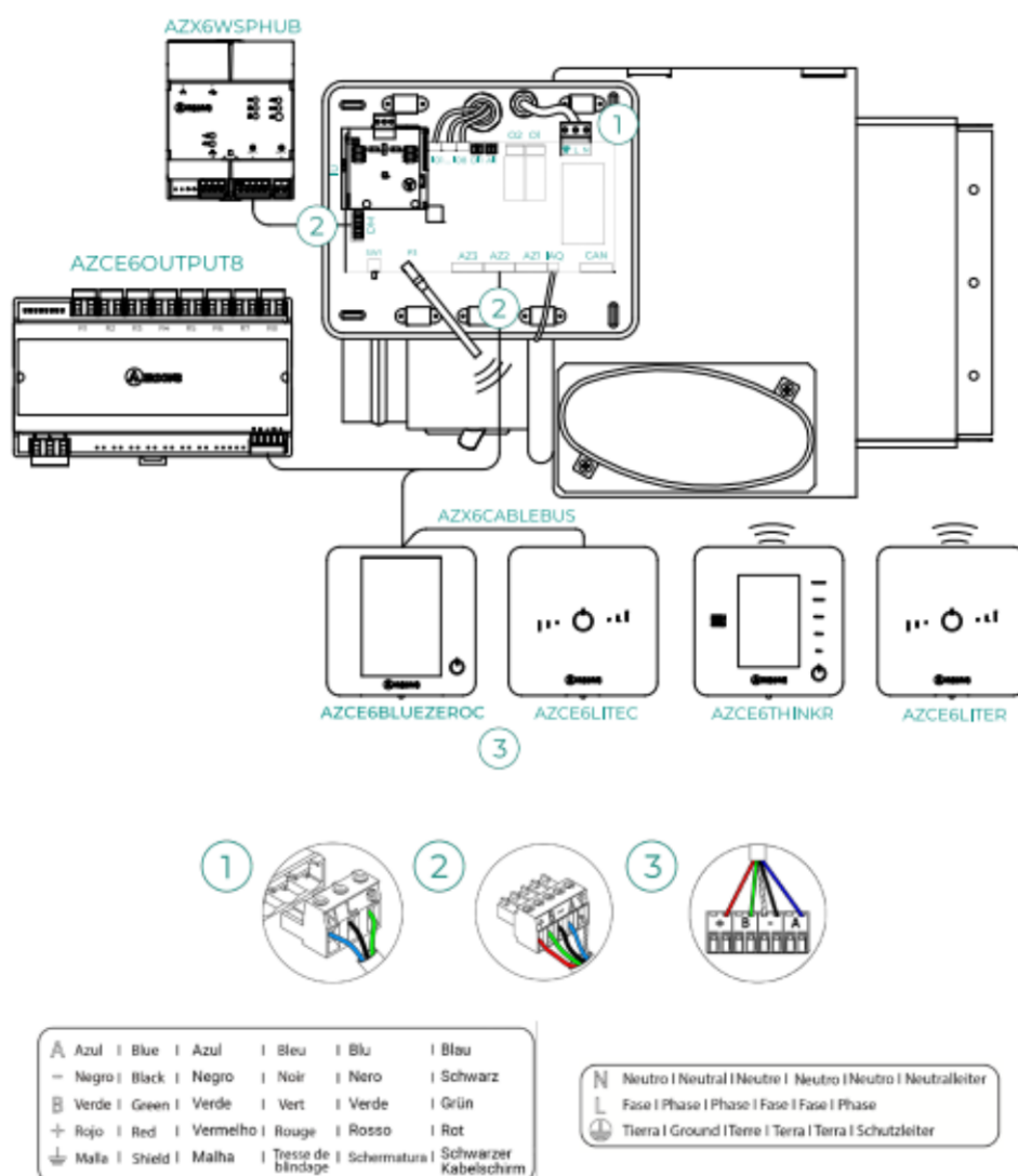
Figure 6 – Schéma d'exemple d'installation n°2 – modèle AZE26
