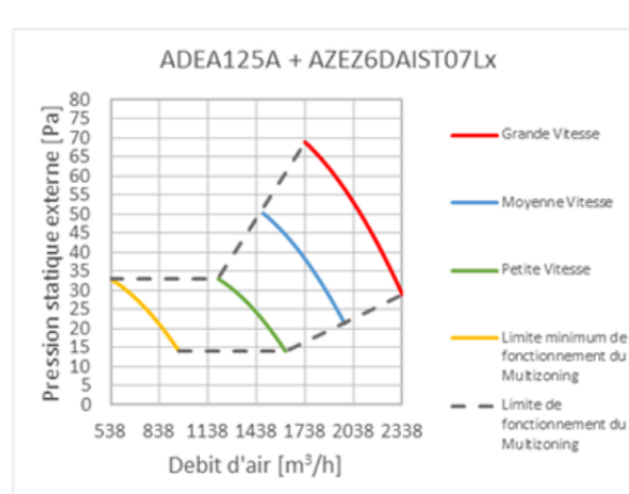
Figure 12 – Unité intérieure ADEA125A Courbes débit/pression
