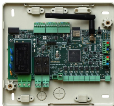
Figure 4a – Contrôleur central de type AZXXXCB1MOTY
