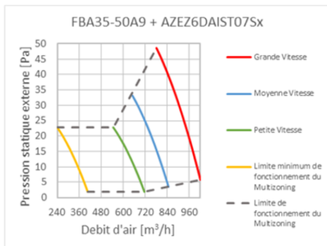
Figure 5 – Unités intérieures FBA35A9 et FBA50A9 Courbes débit/pression
