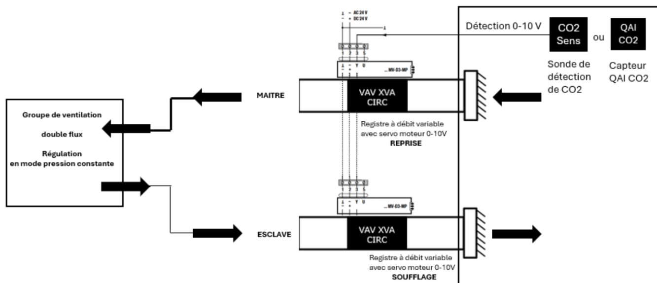
Figure 12b - Pilotage de plusieurs registres à débit variable VAV XVA CIRC ou VAV XVA RECT en fonctionnement « Maître-Esclaves » : cas d'une petite pièce
