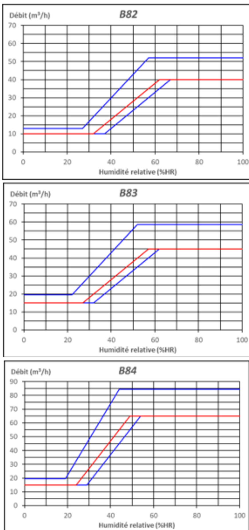
Figure 14 – Caractéristiques hygro-aérauliques des bouches d'extraction type B
