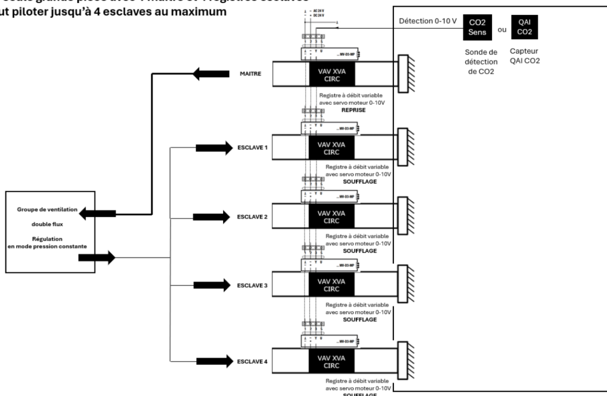
Figure 12d - Pilotage de plusieurs registres à débit variable VAV XVA CIRC ou VAV XVA RECT en fonctionnement « Maître-Esclaves » : cas d'une grande pièce avec 1 maître et 4 registres esclaves (max)
