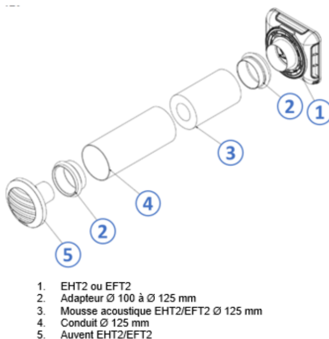
Figure 21c – Mise en œuvre des entrées d'air EHT² ou EFT² en conduit Ø 125 mm L 300 mm
