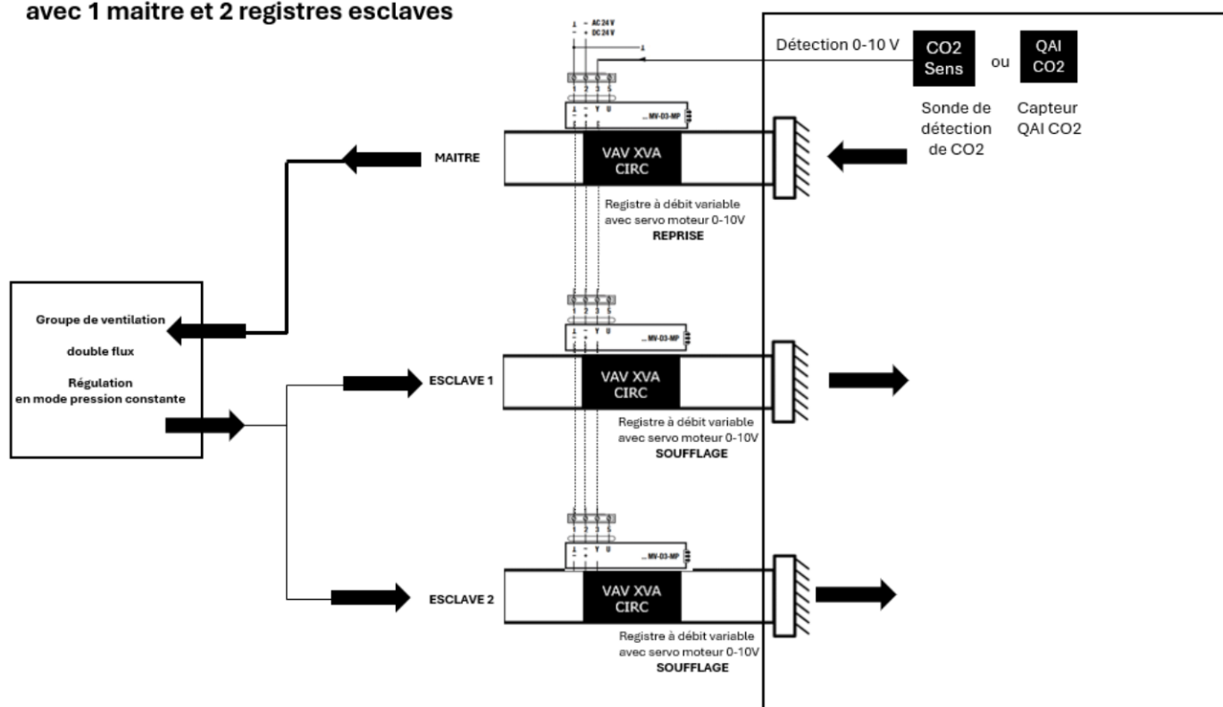
Figure 12c - Pilotage de plusieurs registres à débit variable VAV XVA CIRC ou VAV XVA RECT en fonctionnement « Maître-Esclaves » : cas d'une grande pièce avec 1 maître et 2 registres esclaves
