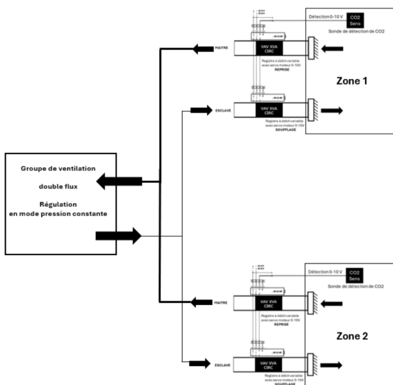
Figure 4 - Cas 2 : branche pilotée par le Registre à débit variable VAV XVA CIRC ou VAV XVA RECT – CO 2
