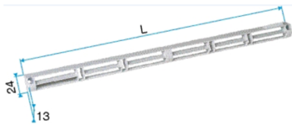
Auvent standard pour mini EA 30
