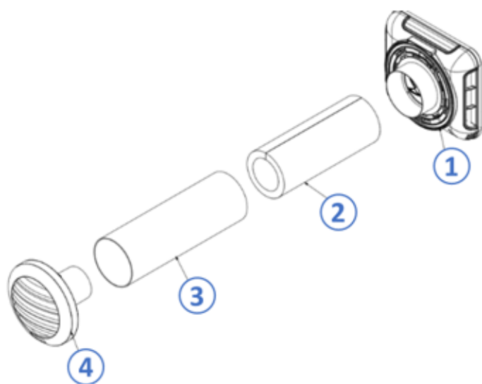
Figure 21a – Mise en œuvre des entrées d'air EHT 2 ou EFT 2 sans mousse Ø 100 mm L 300 mm
