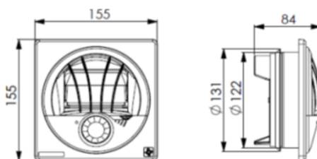
Figure 6 - Terminal « TDA »
