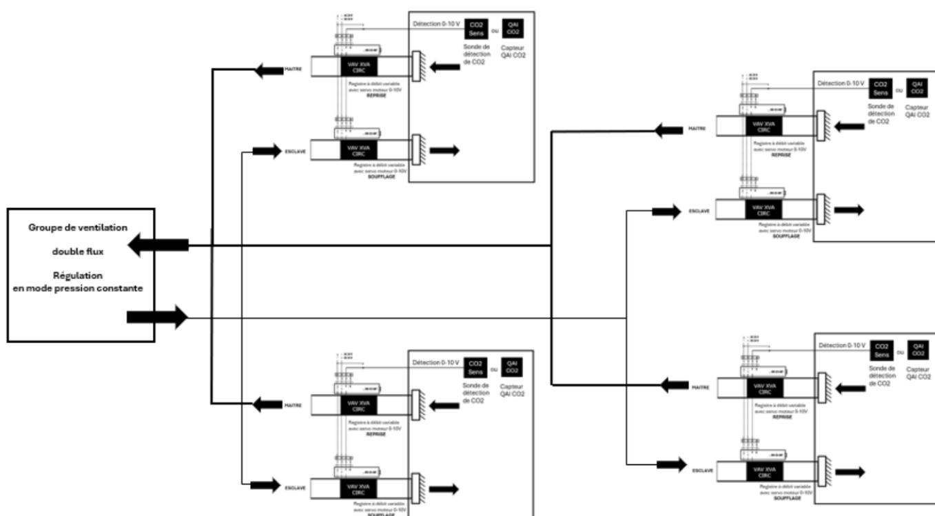
Figure 12e - Pilotage de plusieurs registres à débit variable VAV XVA CIRC ou VAV XVA RECT en fonctionnement « Maître-Esclaves » : cas de 4 pièces distinctes
